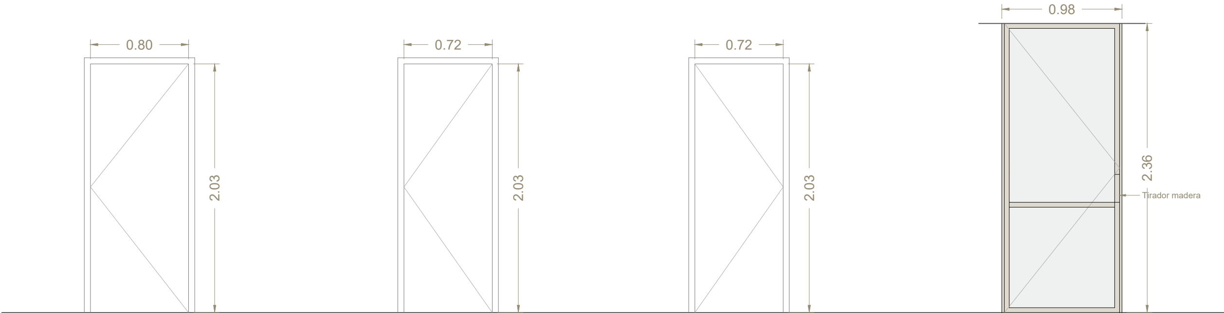
PE Panelado en lacado blanco de puerta existente Cambio de herrajes y manivela P01 Puerta abatible Acabado lacado blanco Con condena Herrajes y manivela metálicos blancos a definir
