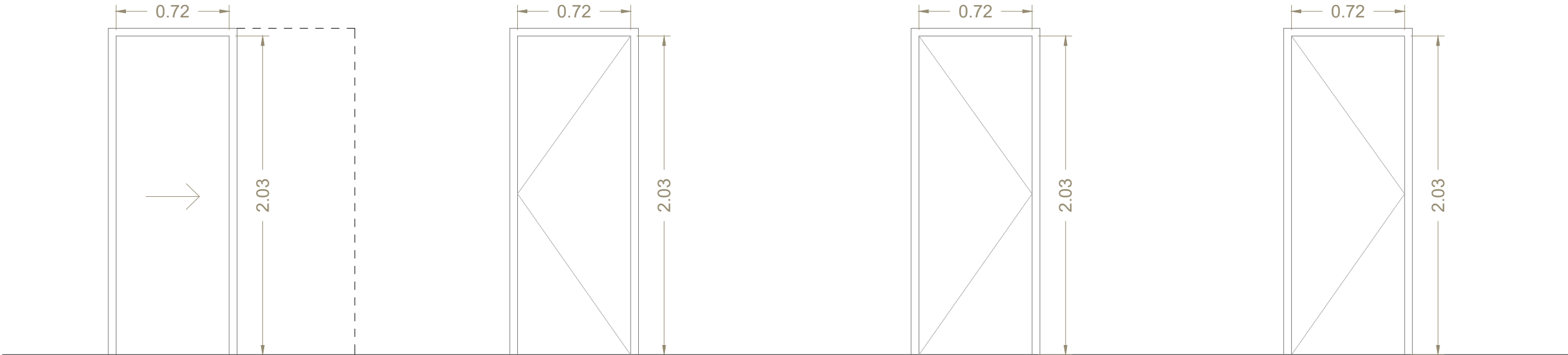
P04 Puerta corerdera Acabado lacado blanco Con condena Uñero metálico blanco a definir
