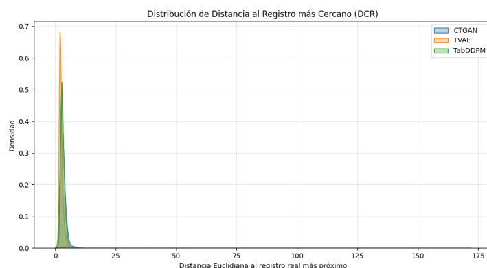
Figura 4: Distribución probabilística de las distancias euclidianas (DCR) frente al paciente biológico más cercano. La total ausencia de solapamiento en el origen (valor cero) descarta el fenómeno de memorización fotográfica.
