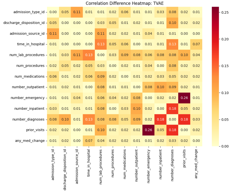
Figura 2: Mapa residual de Diferencia de Correlación para TVAE. La regularización bayesiana difumina agresivamente las fronteras, destruyendo la señal minoritaria.
