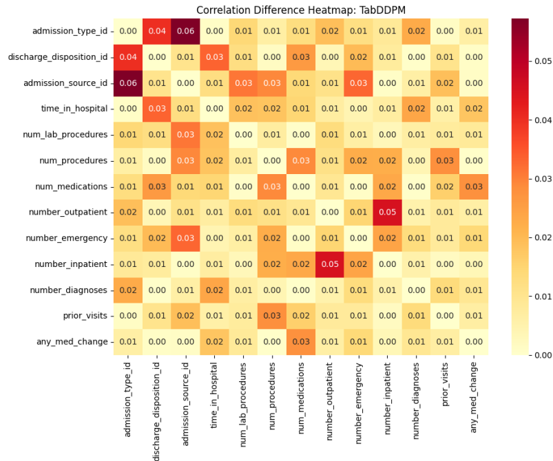
Figura 3: Mapa residual de Diferencia de Correlación para TabDDPM. La pureza de los tonos blancos certifica una asombrosa reconstrucción de la matriz covariante original.
