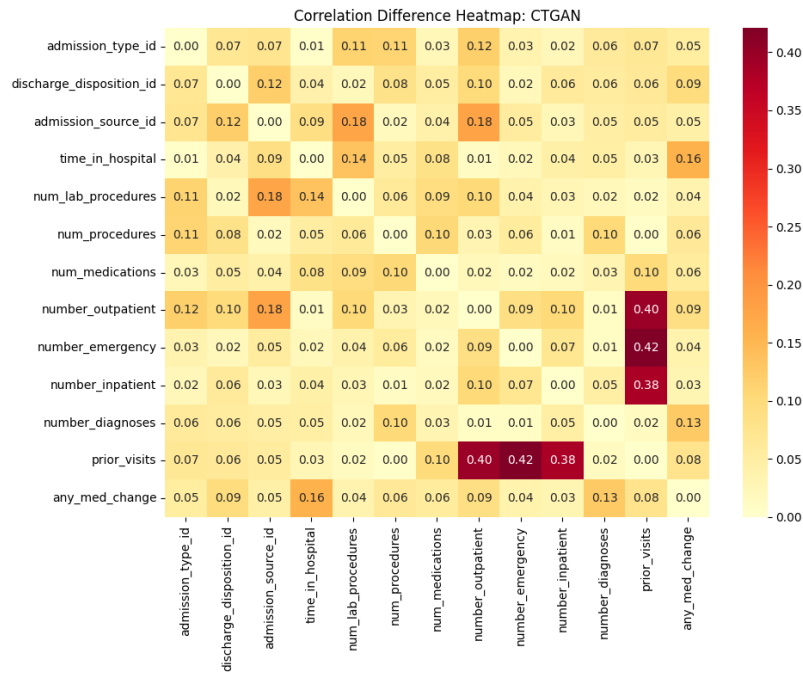
Figura 1: Mapa residual de Diferencia de Correlación para CTGAN. Obsérvense las severas invenciones espurias (tonos rojos) causadas por la inestabilidad adversarial.
