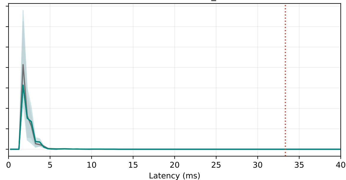
WMM on: CS5 / AC_VI
