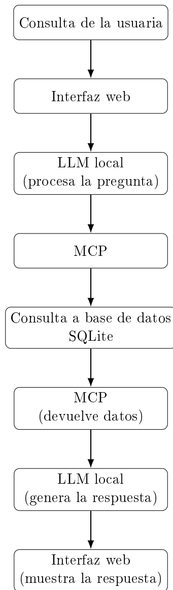
Figura 5.10: Flujo de interacción con la interfaz web y su conexión con el LLM local y la base de datos SQLite.
