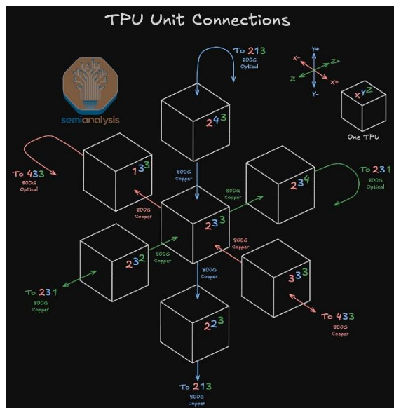
谷歌TPU方案拓扑图
