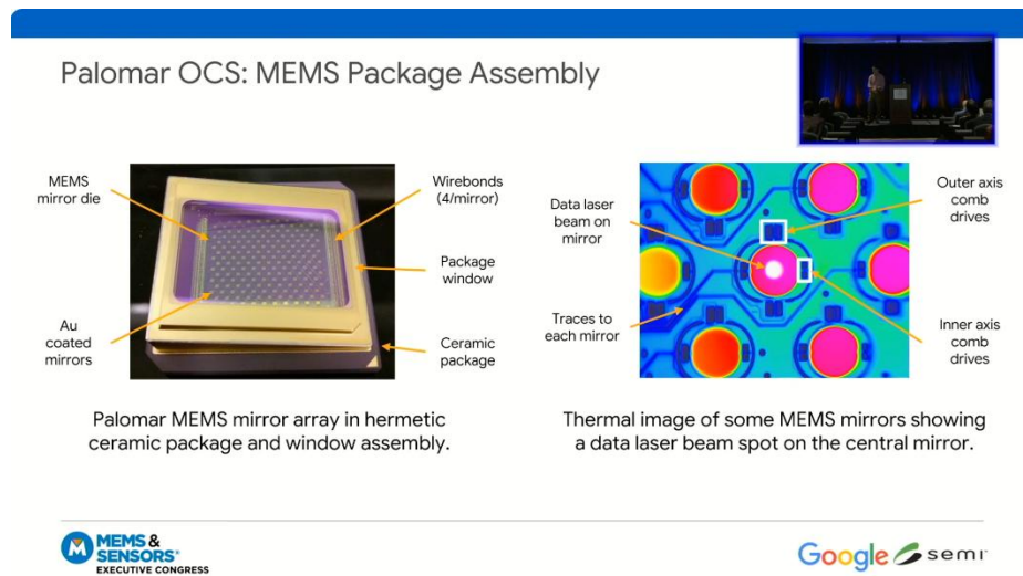
MEMS微振镜
