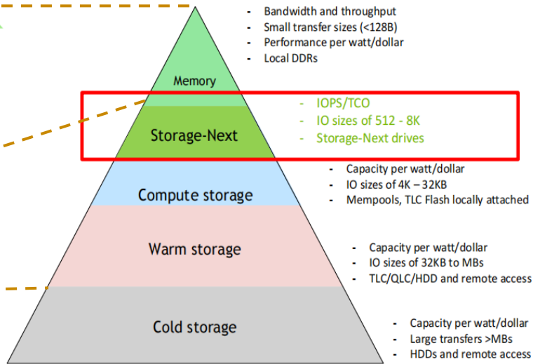
数据层级结构示意图
