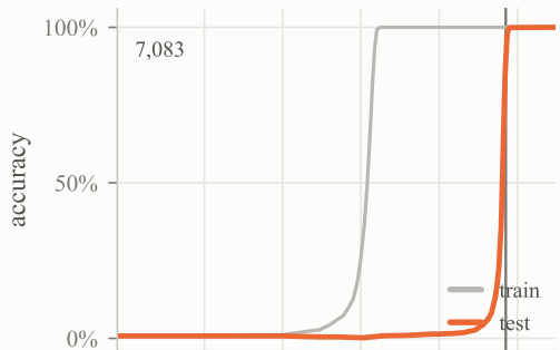
(a^2 + ab + b^2) \bmod p p=113
