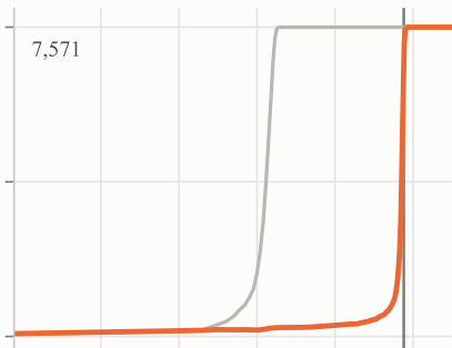
(a * b) \bmod p p=113
