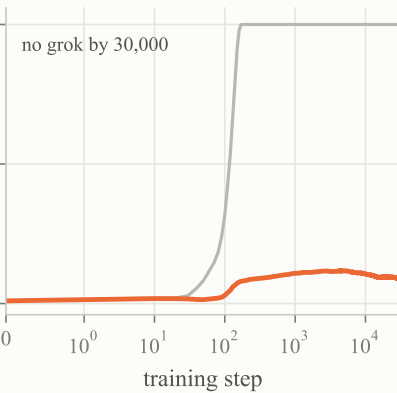
(a^2 + ab + b^2) \bmod p p=109
