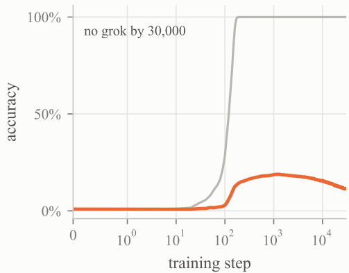
(a^2 + ab + b^2) \bmod p p=113
