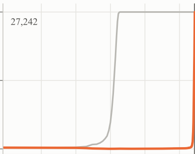
(a^2 + ab + b^2) \bmod p p=109
