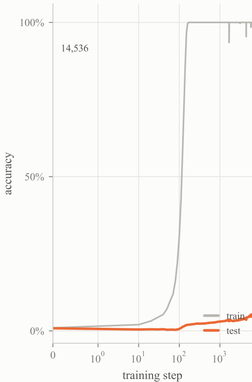
(a + b) \bmod p p=113
