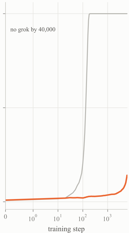
(a * b) \bmod p p=113
