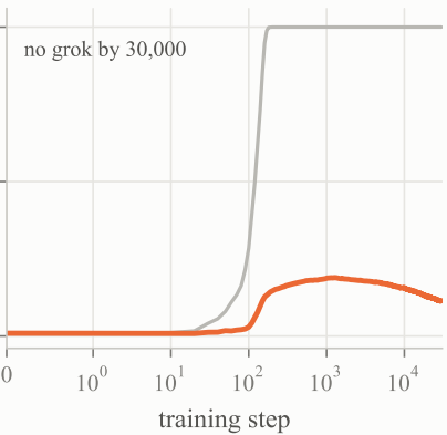
(a^2 + ab + b^2) \bmod p p=113
