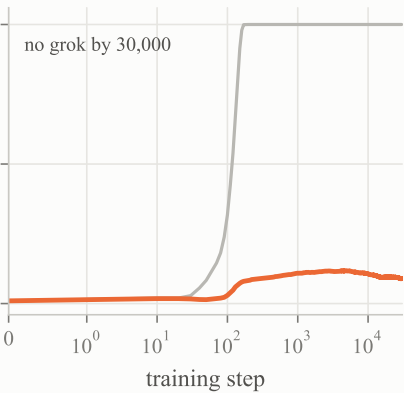
(a^2 + ab + b^2) \bmod p p=109
