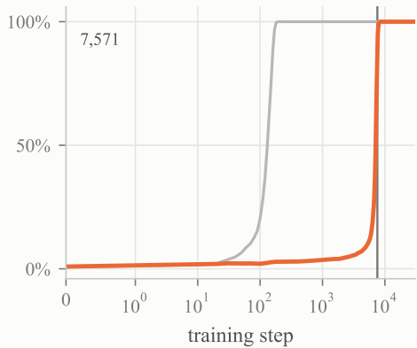
(a * b) \bmod p p=113
