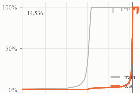
(a * b) \bmod p p=113
