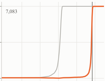
(a^2 + ab + b^2) \bmod p p=113
