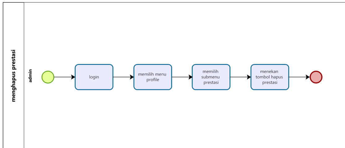
Gambar 19 BPMN Menghapus Prestasi Sekolah
