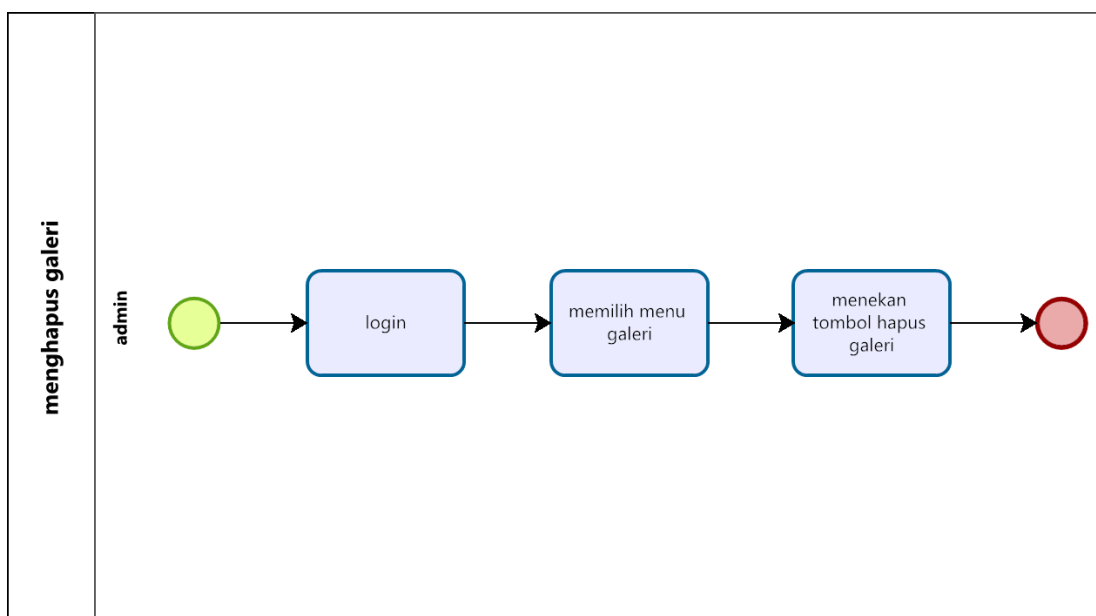
Gambar 25 BPMN Menghapus Galeri
