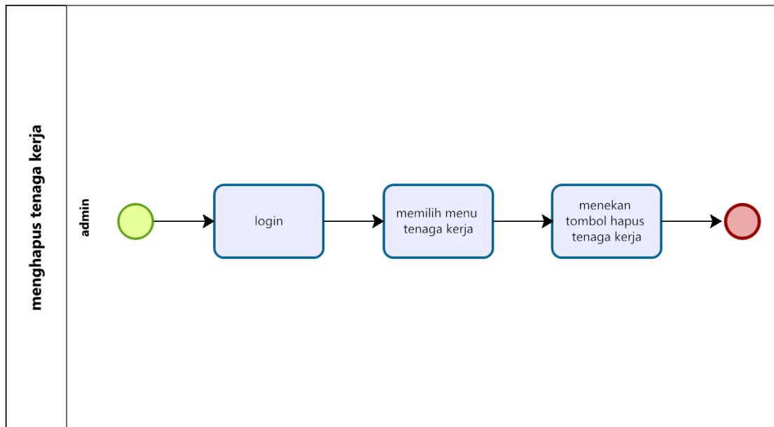
Gambar 22 BPMN Menghapus Tenaga Kerja
