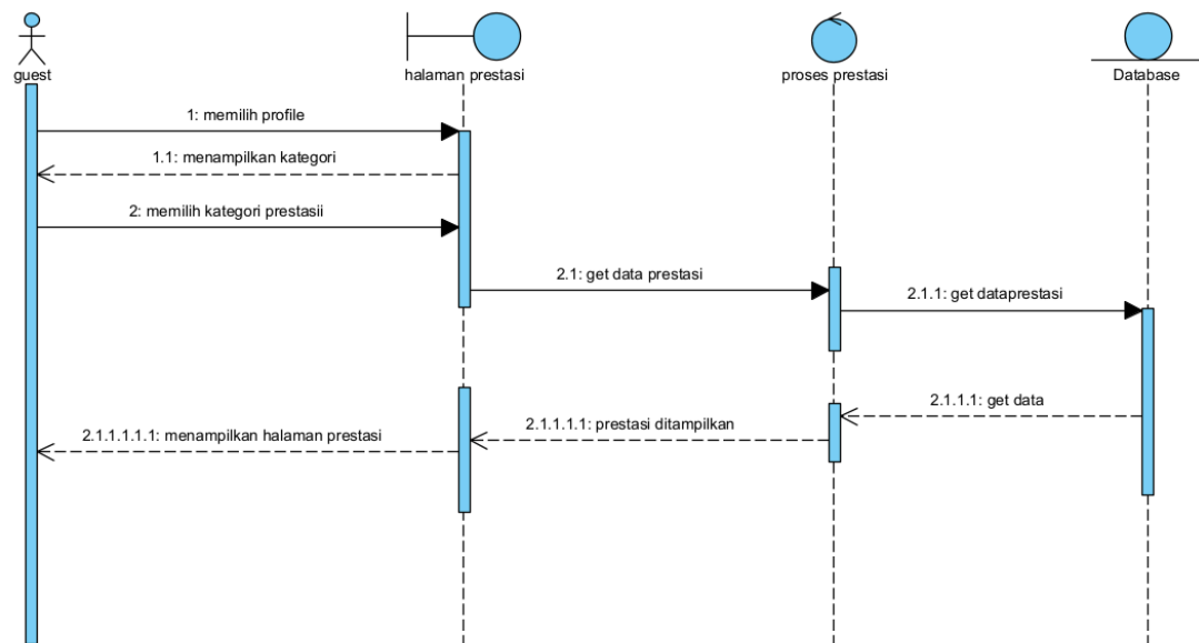
Gambar 40 Sequence Diagram Melihat Prestasi
