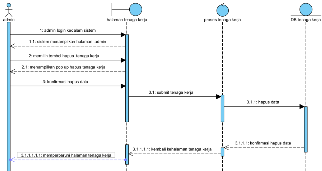
Gambar 63 Sequence Diagram Menghapus Tenaga Kerja
