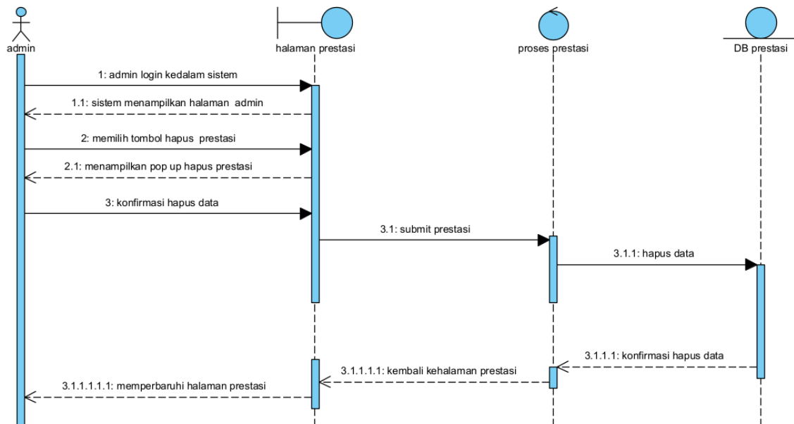
Gambar 61 Sequence Diagram Menghapus Prestasi
