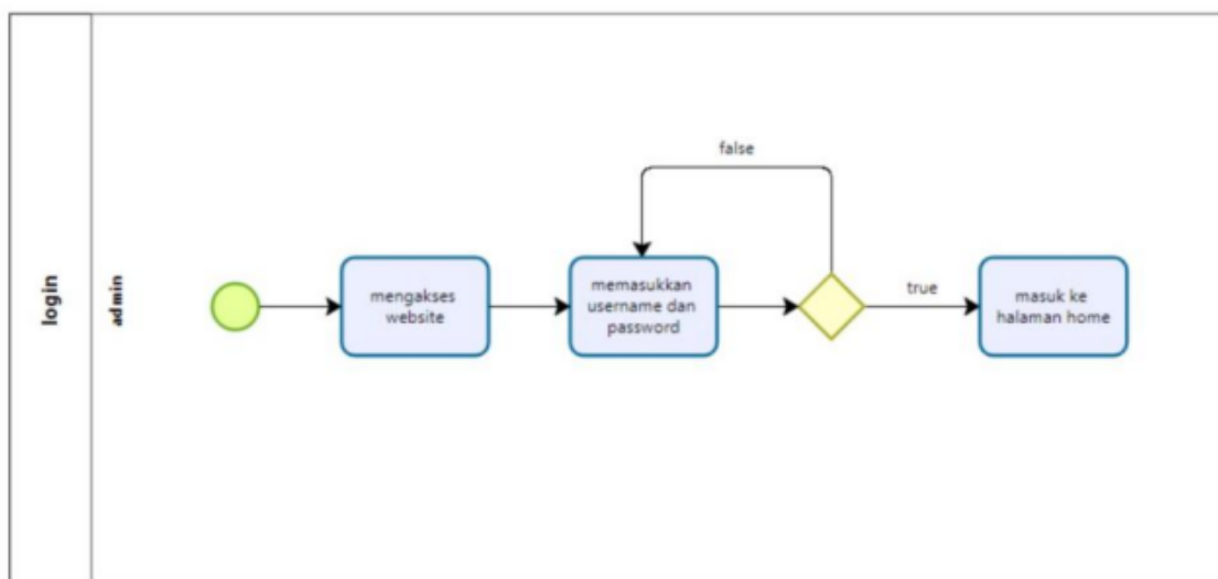
Gambar 3 BPMN Login
