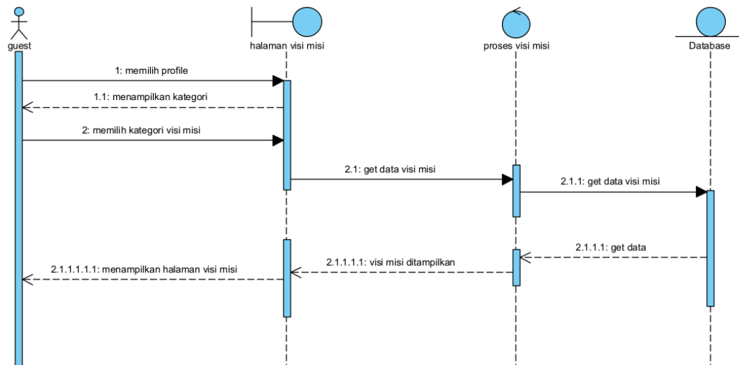
Gambar 39 Sequence Diagram Melihat Visi-misi
