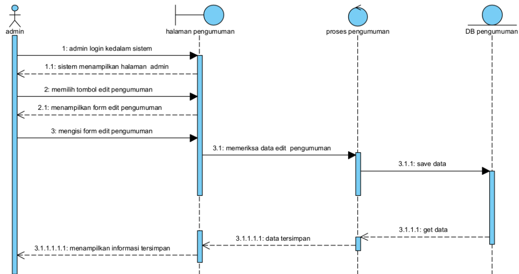
Gambar 67 Sequence Diagram Mengedit Pengumuman
