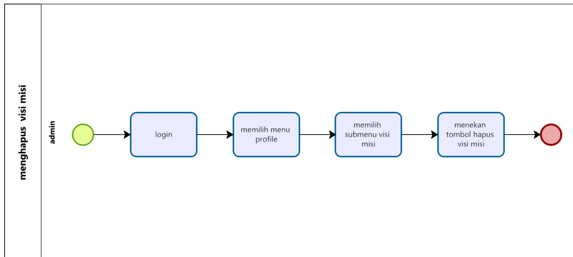
Gambar 15 BPMN Menghapus visi misi
