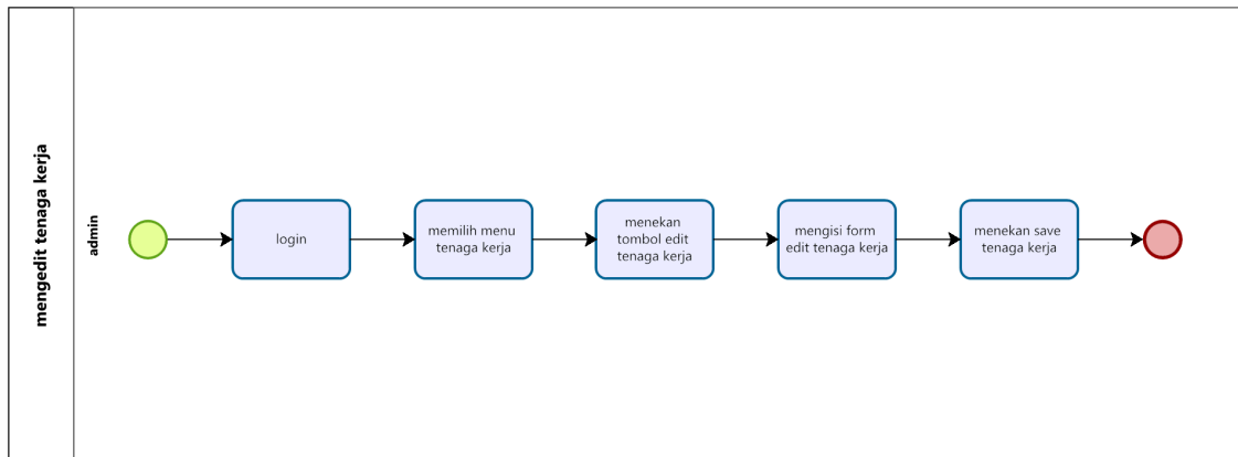
Gambar 21 BPMN Mengedit Tenaga Kerja
