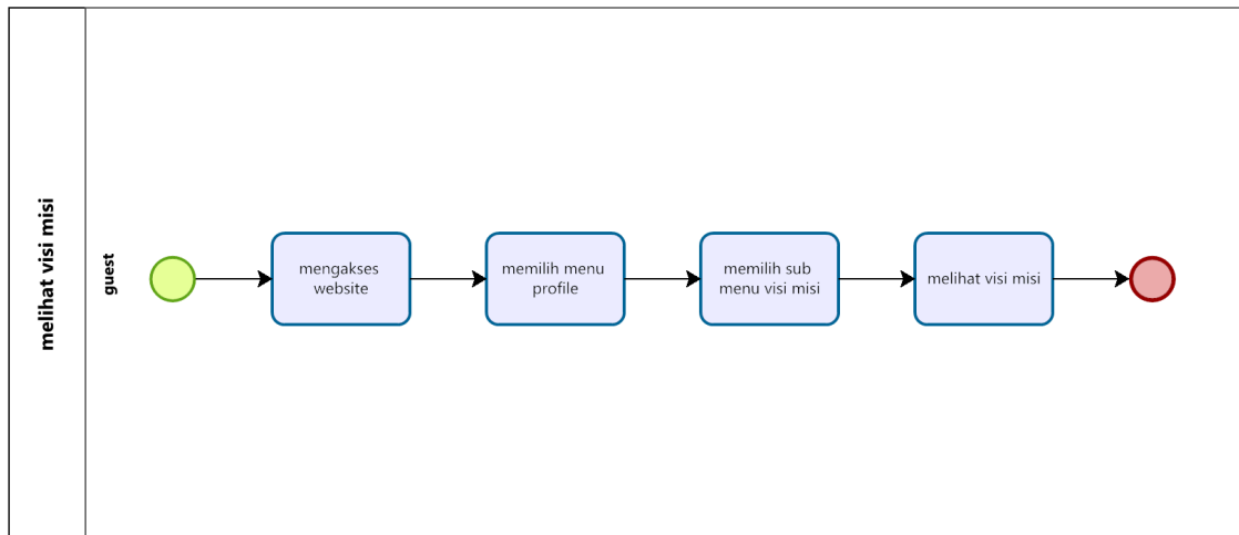
Gambar 4 BPMN Melihat Visi Misi Pada Guest
