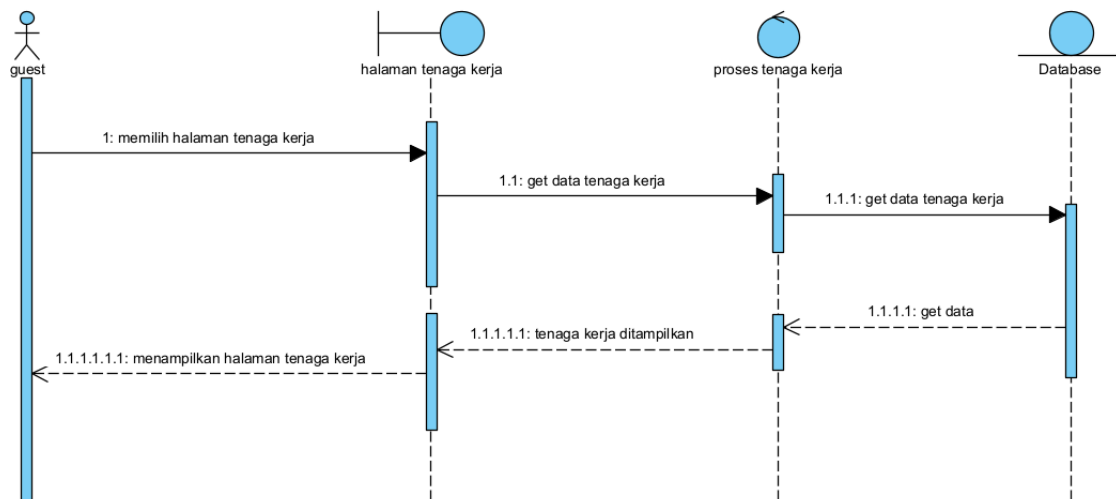
Gambar 44 Sequence Diagram Melihat Tenaga Kerja
