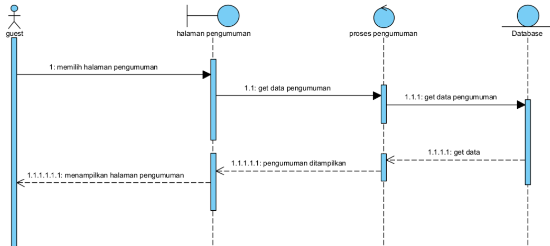
Gambar 43 Sequence Diagram Melihat Pengumuman
