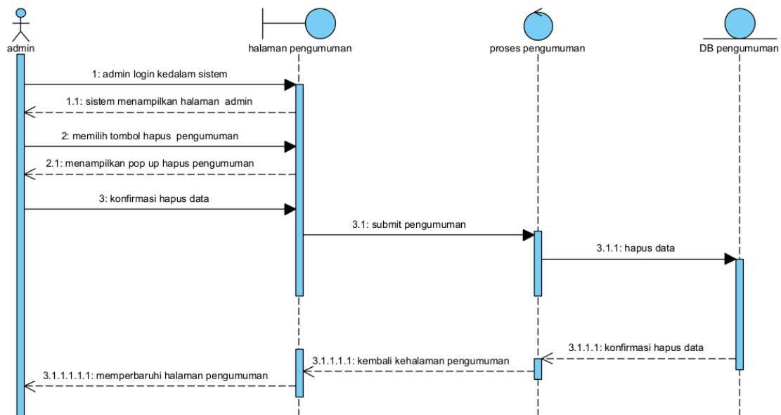
Gambar 64 Sequence Diagram Menghapus Pengumuman
