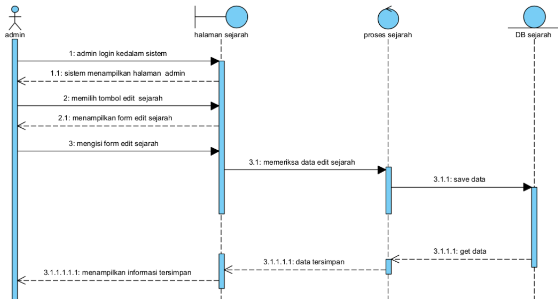
Gambar 57 Sequence Diagram Mengedit sejarah
