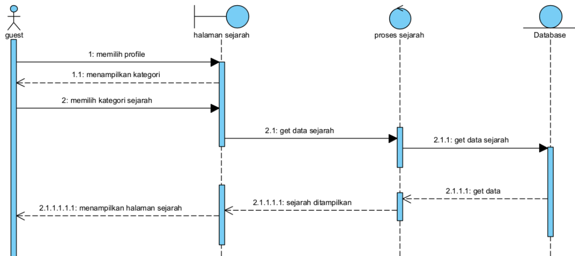
Gambar 41 Sequence Diagram Melihat Sejarah
