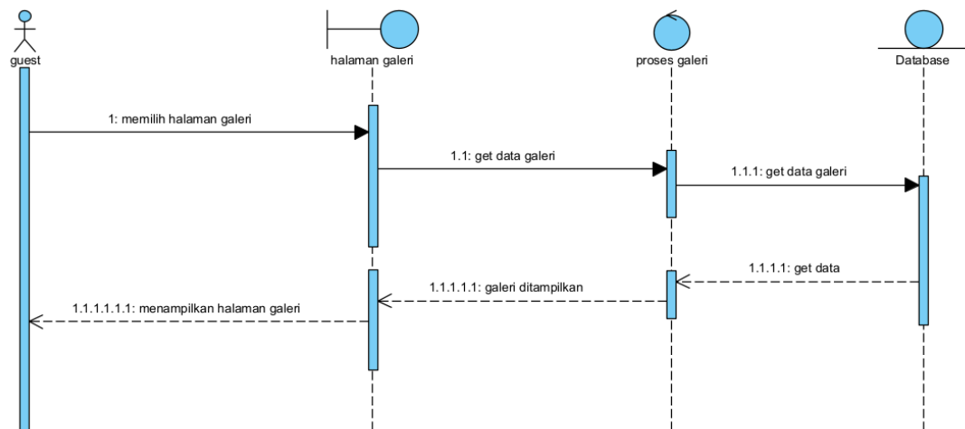
Gambar 42 Sequence Diagram Melihat Galeri
