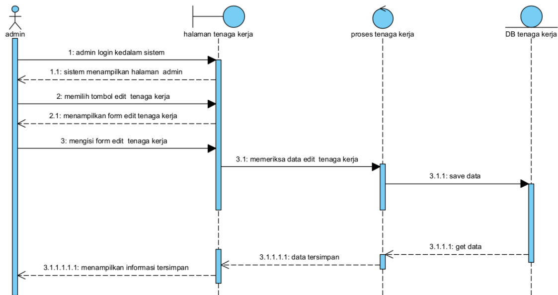
Gambar 54 Sequence Diagram Mengedit Tenaga Kerja
