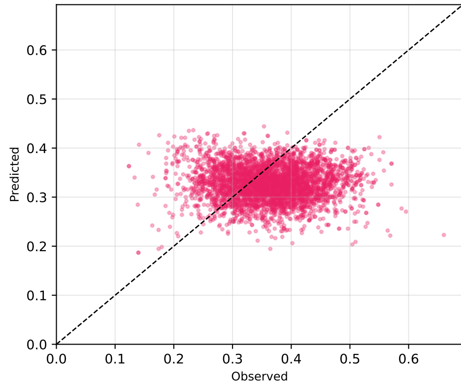
Ibuprofen RMSE=0.0830
