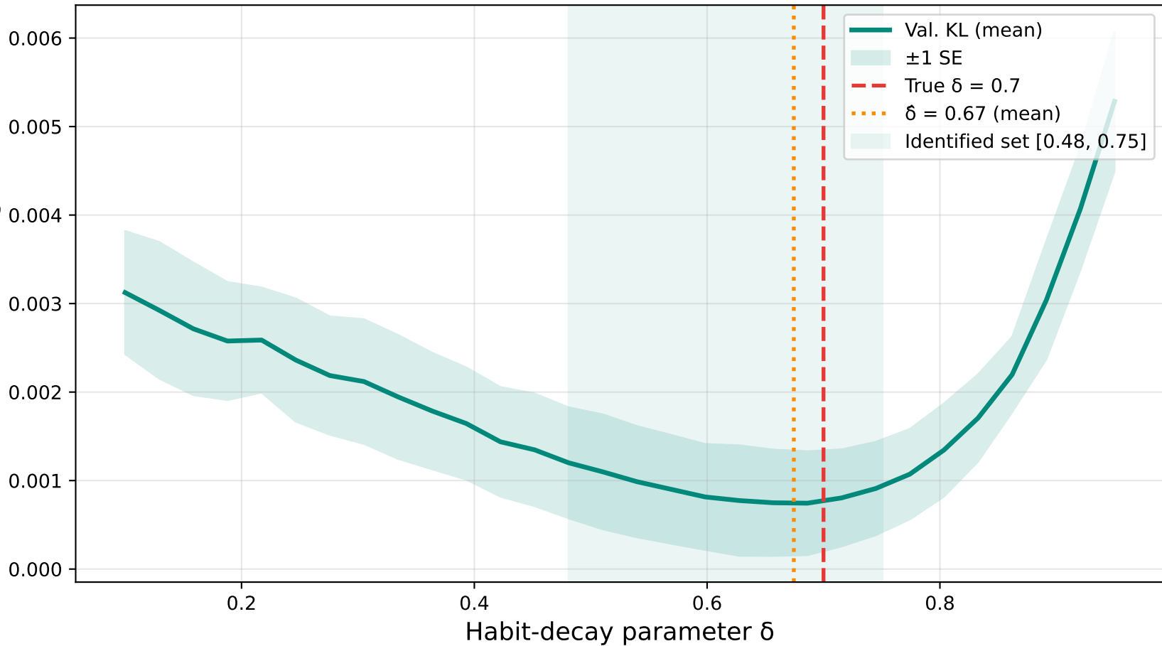
Validation KL divergence
