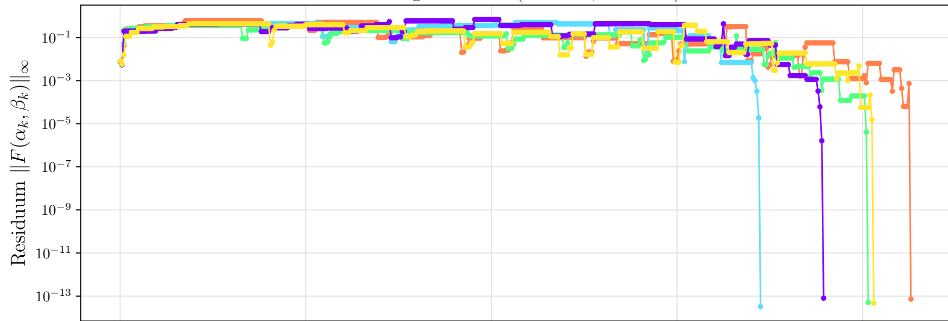
Konvergenzverlauf ( n = 256, m = 256 )
