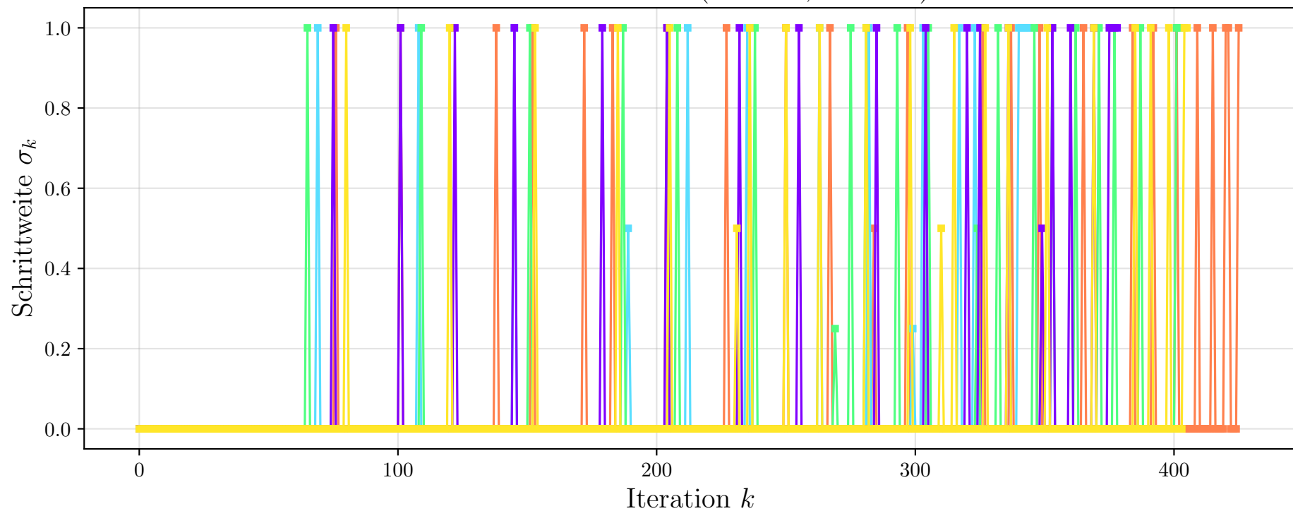
Schrittweitenverlauf ( n = 256, m = 256 )
