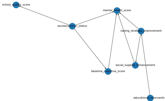
Statistical DAG
