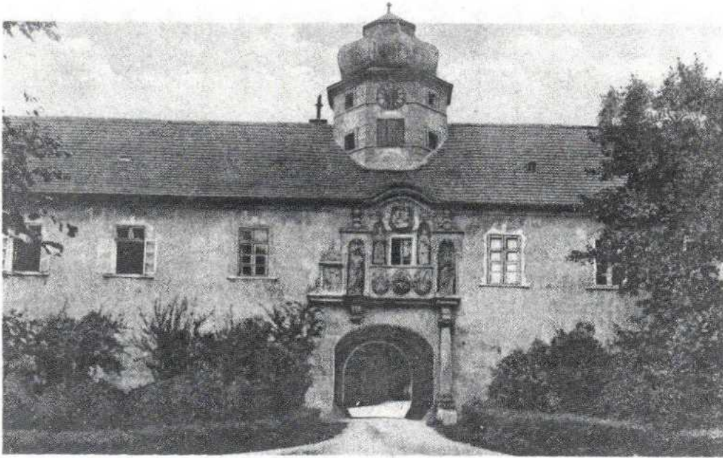
Oberglogau, Schloßportal
