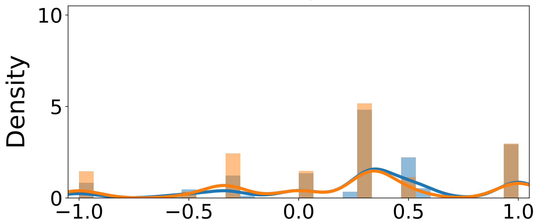
Prompt 3
