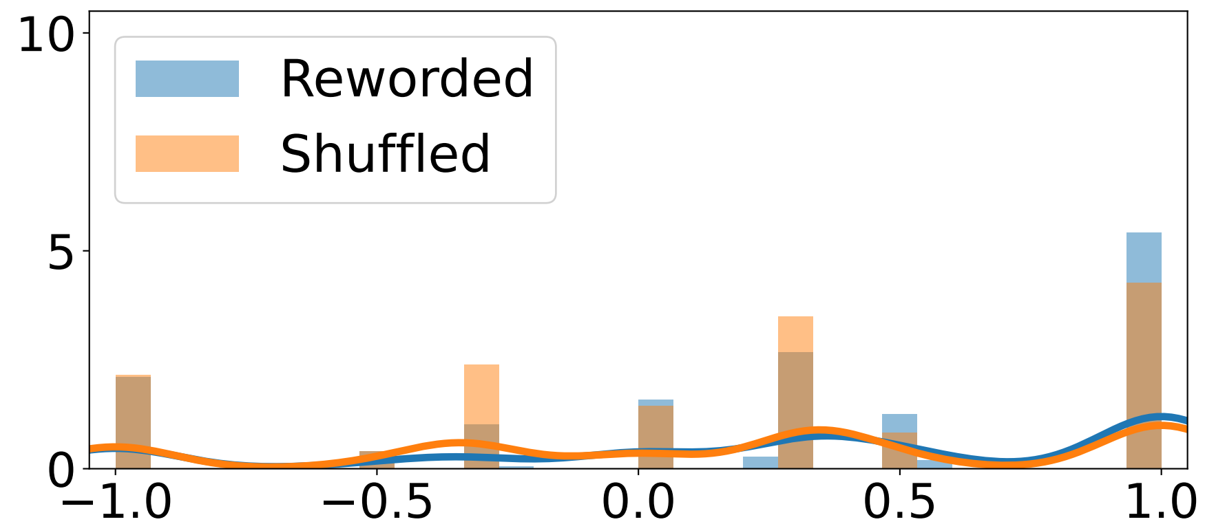
Prompt 4
