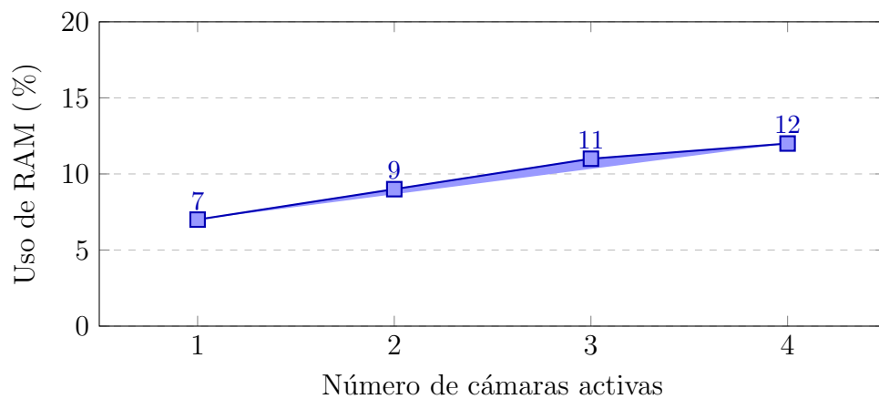
Figura 5.4: Consumo de RAM de voctocore en función del número de cámaras activas. La RAM crece de forma sublineal al aumentar las fuentes, ya que el pipeline GStreamer comparte buffers internos entre ellas.
