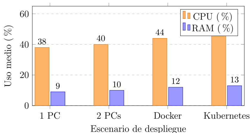
Figura 5.6: Consumo medio de CPU y RAM de voctocore por escenario de despliegue, con cuatro fuentes activas.
