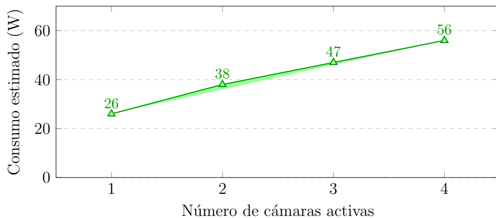
Figura 5.5: Consumo energético estimado en función del número de cámaras activas, calculado a partir del porcentaje de CPU y la TDP del procesador (45 W TDP, i7-8750H).
