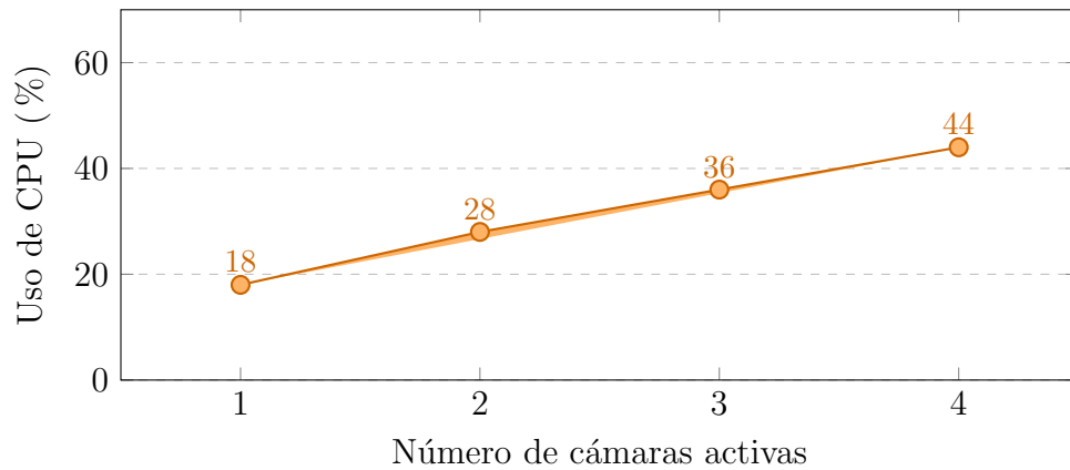
Figura 5.3: Consumo de CPU de voctocore en función del número de cámaras activas (mediana de entradas STATE, sesión de 5 min, 1080p25, Docker Compose).
