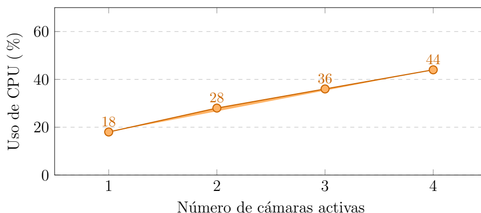
Figura 5.3: Consumo de CPU de voctocore en función del número de cámaras activas.
