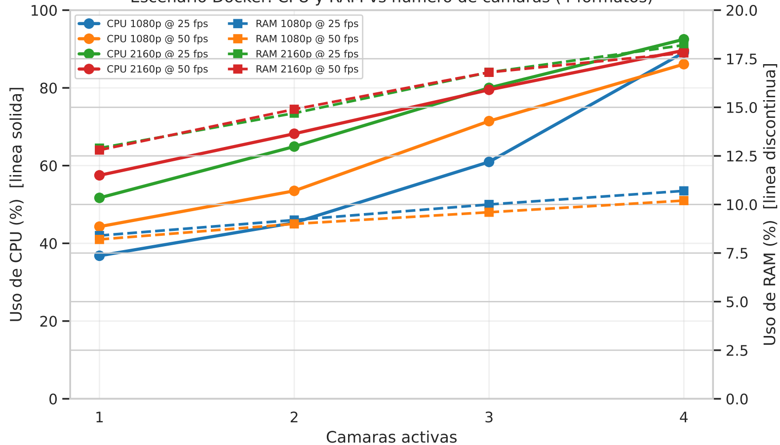
Escenario Docker: CPU y RAM vs numero de camaras (4 formatos)
