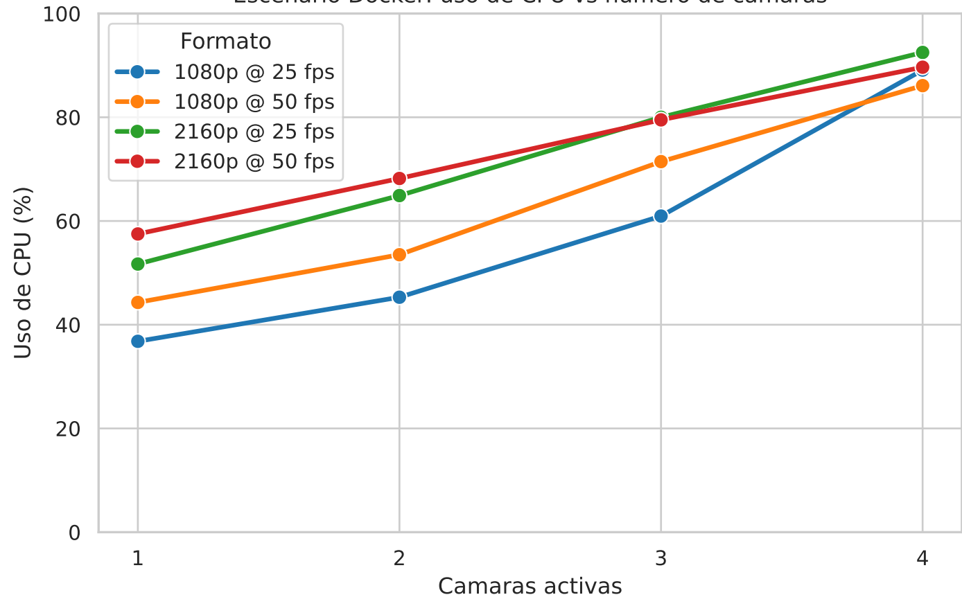
Escenario Docker: uso de CPU vs numero de camaras
