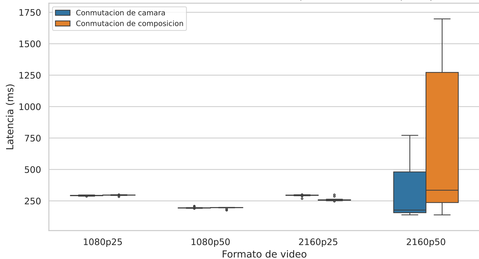
Escenario Docker: latencia de conmutacion por formato (n=100 por caja)
