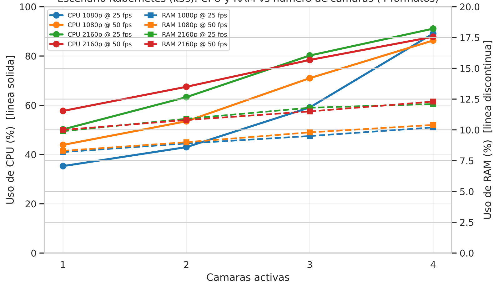
Escenario Kubernetes (k3s): CPU y RAM vs numero de camaras (4 formatos)
