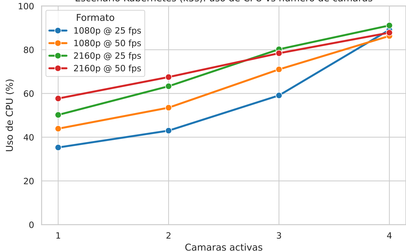
Escenario Kubernetes (k3s): uso de CPU vs numero de camaras
