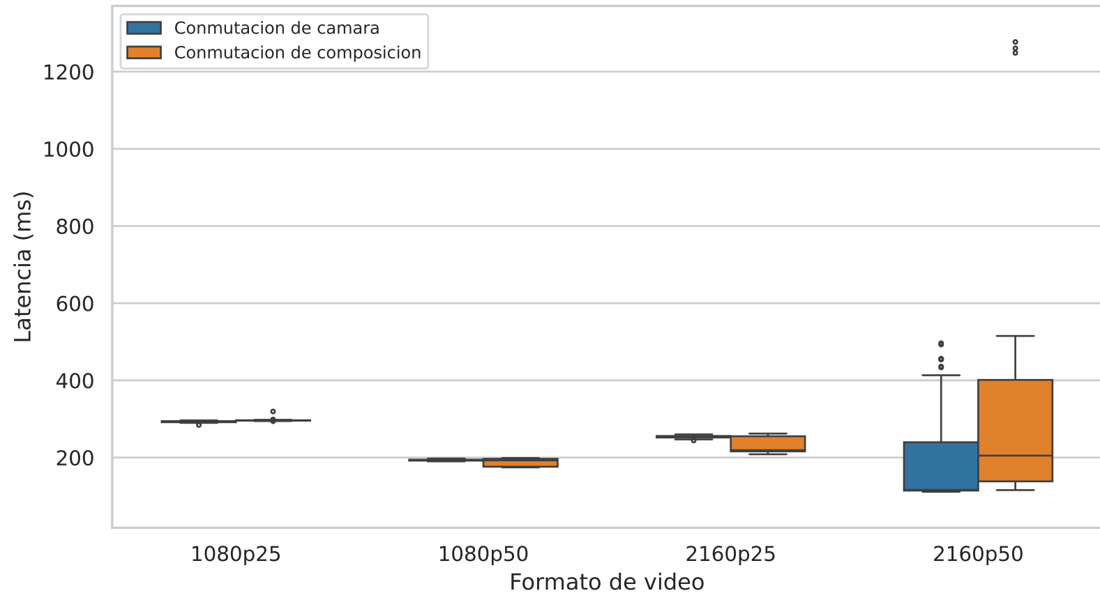
Escenario Kubernetes (k3s): latencia de conmutacion por formato (n=100 por caja)
