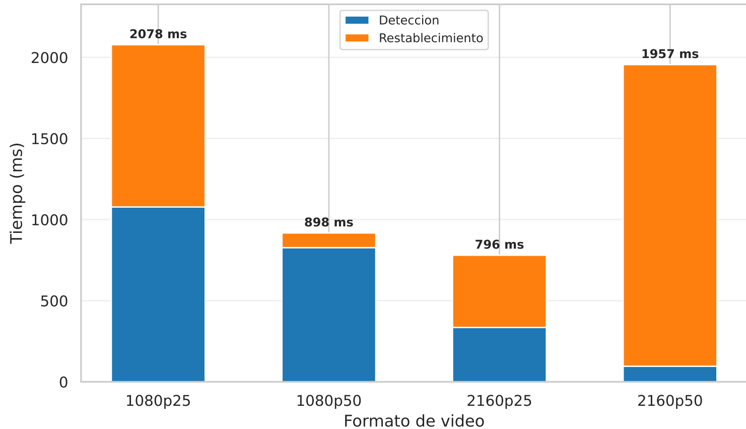
Escenario Kubernetes (k3s): MTTR de recuperacion de camara (deteccion + restablecimiento)
