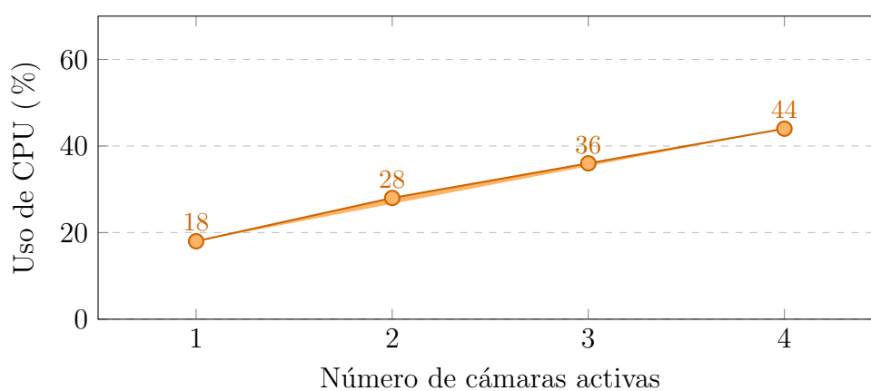
Figura 5.3: Consumo de CPU de voutocore en función del número de cámaras activas.
