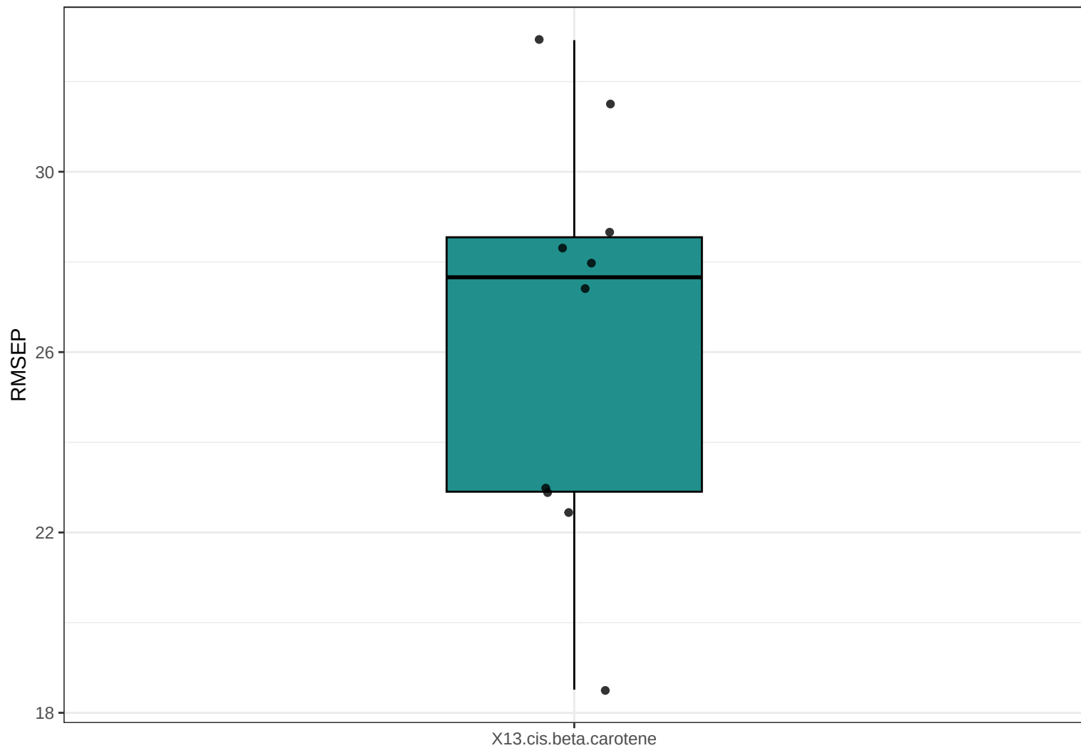
Boxplot RMSEP (PLS) : X13.cis.beta.carotene
