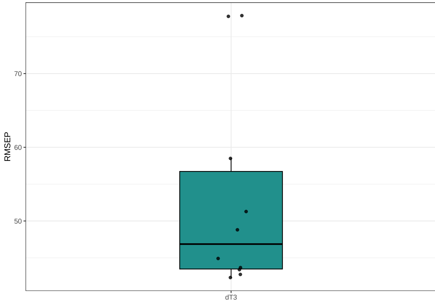
Boxplot RMSEP (PLS) : dT3
