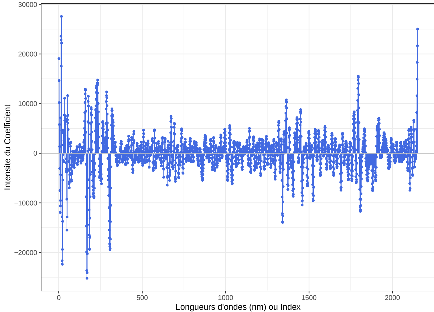
PLS – Vecteur des coefficients : gT3
