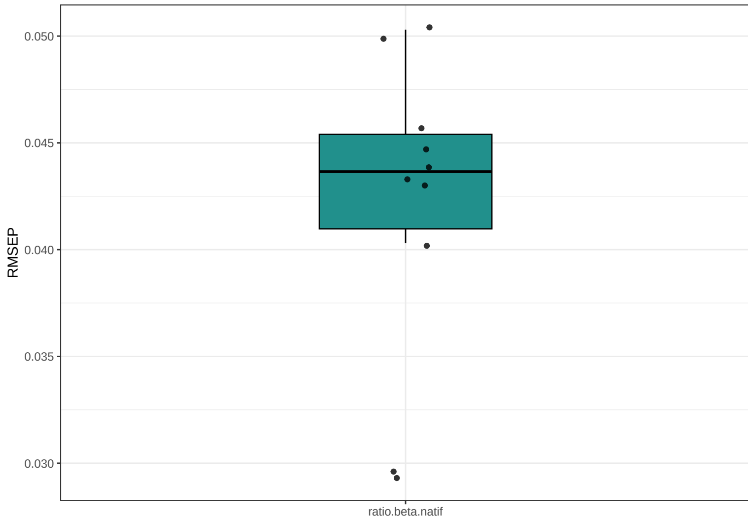
Boxplot RMSEP (PLS) : ratio.beta.natif
