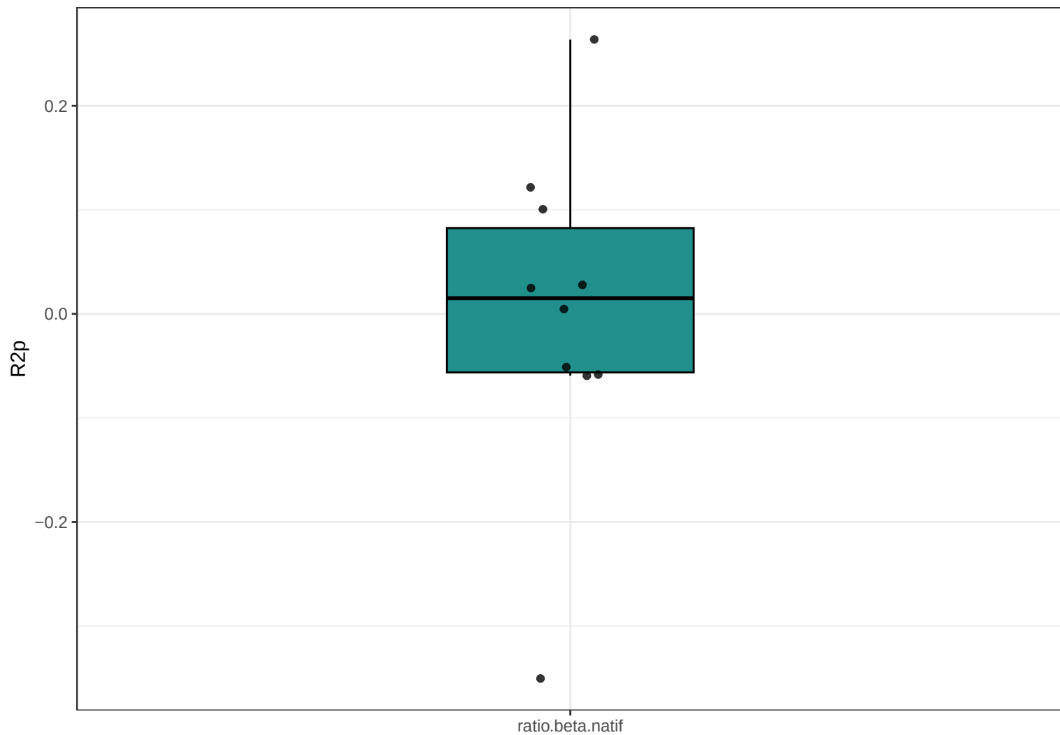
Boxplot R2p (PLS) : ratio.beta.natif
