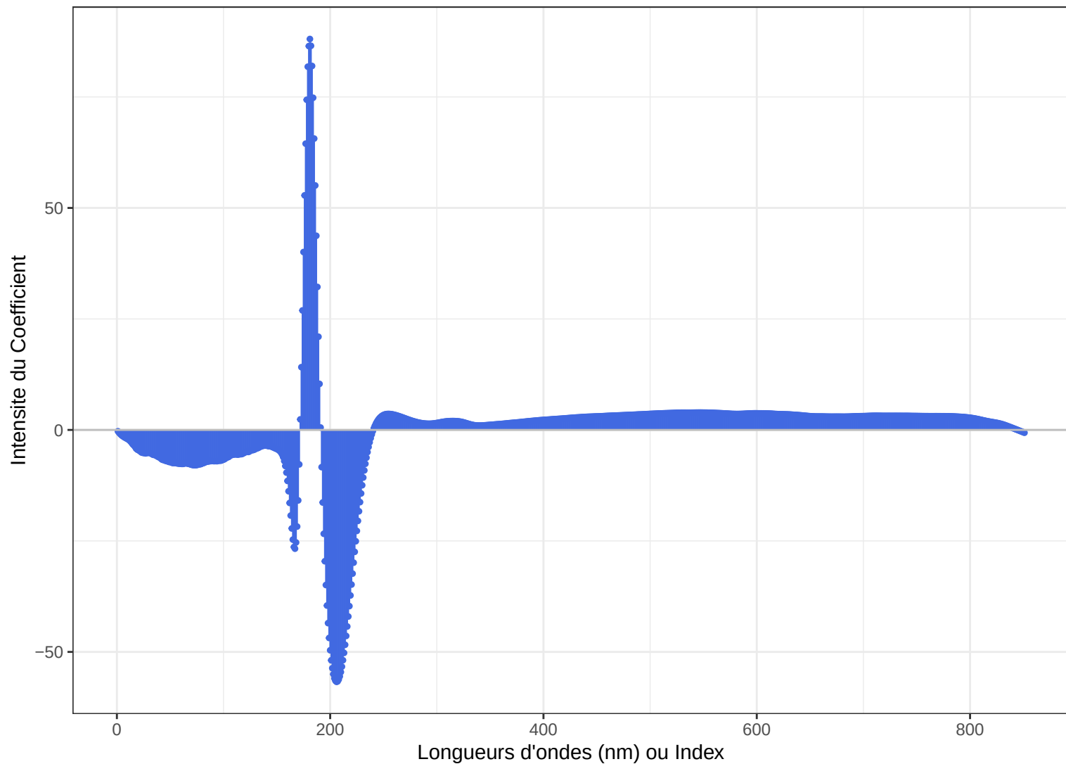
PLS – Vecteur des coefficients : total.trans.carotenes.natif
