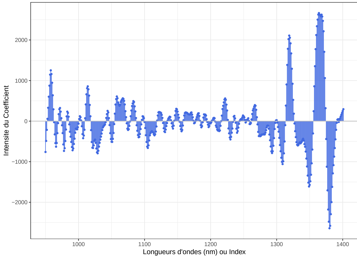
PLS – Vecteur des coefficients : C18.1n9
