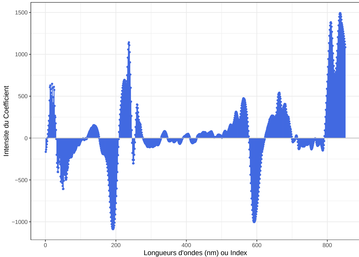
PLS – Vecteur des coefficients : total.beta.carotene
