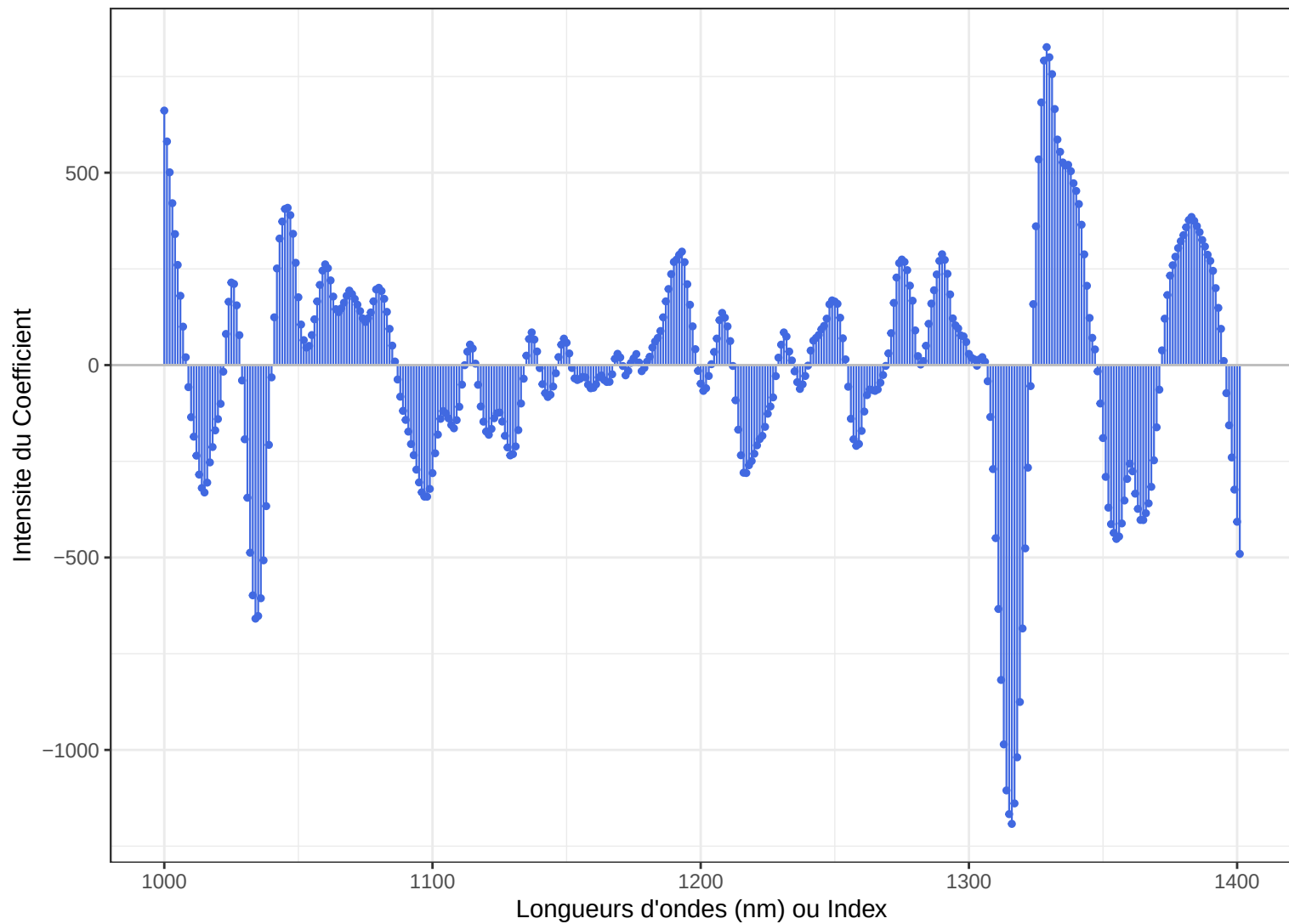
PLS – Vecteur des coefficients : C16.0
