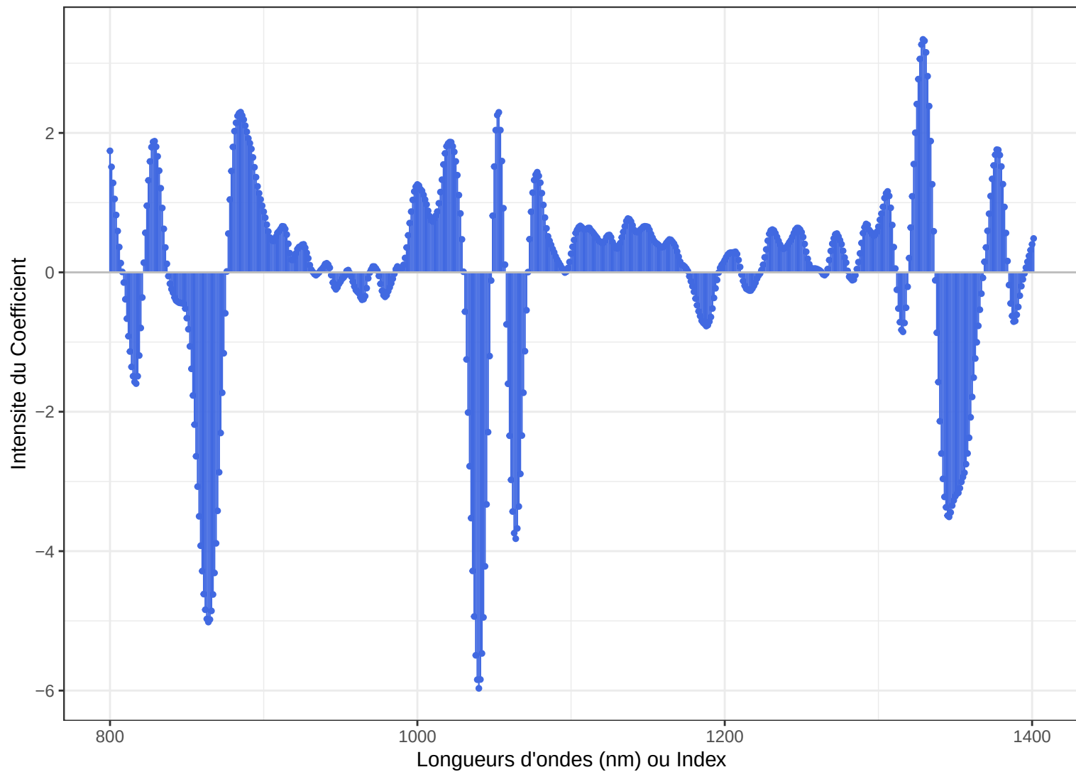
PLS – Vecteur des coefficients : C18.3
