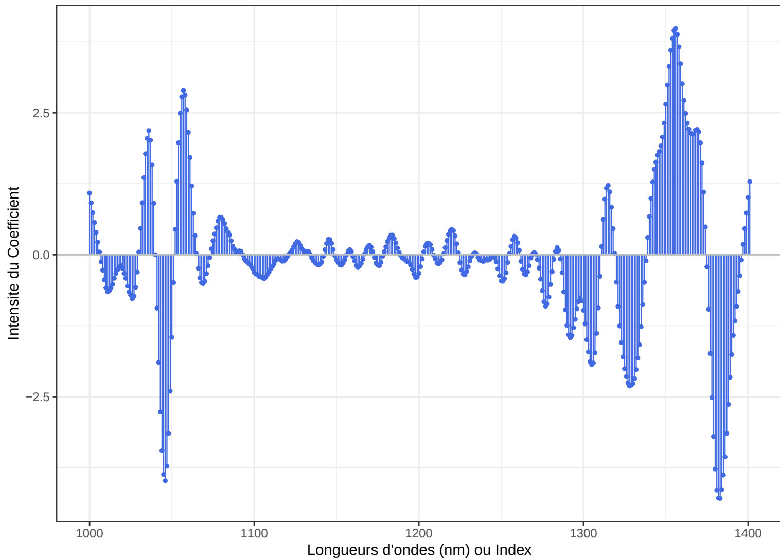
PLS – Vecteur des coefficients : C20.0
