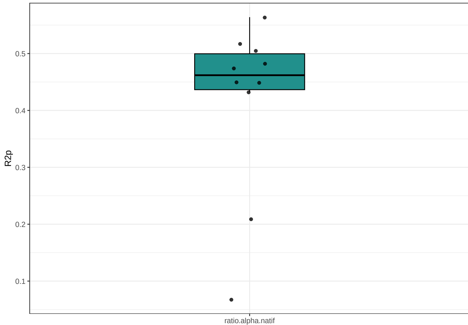
Boxplot R2p (PLS) : ratio.alpha.natif
