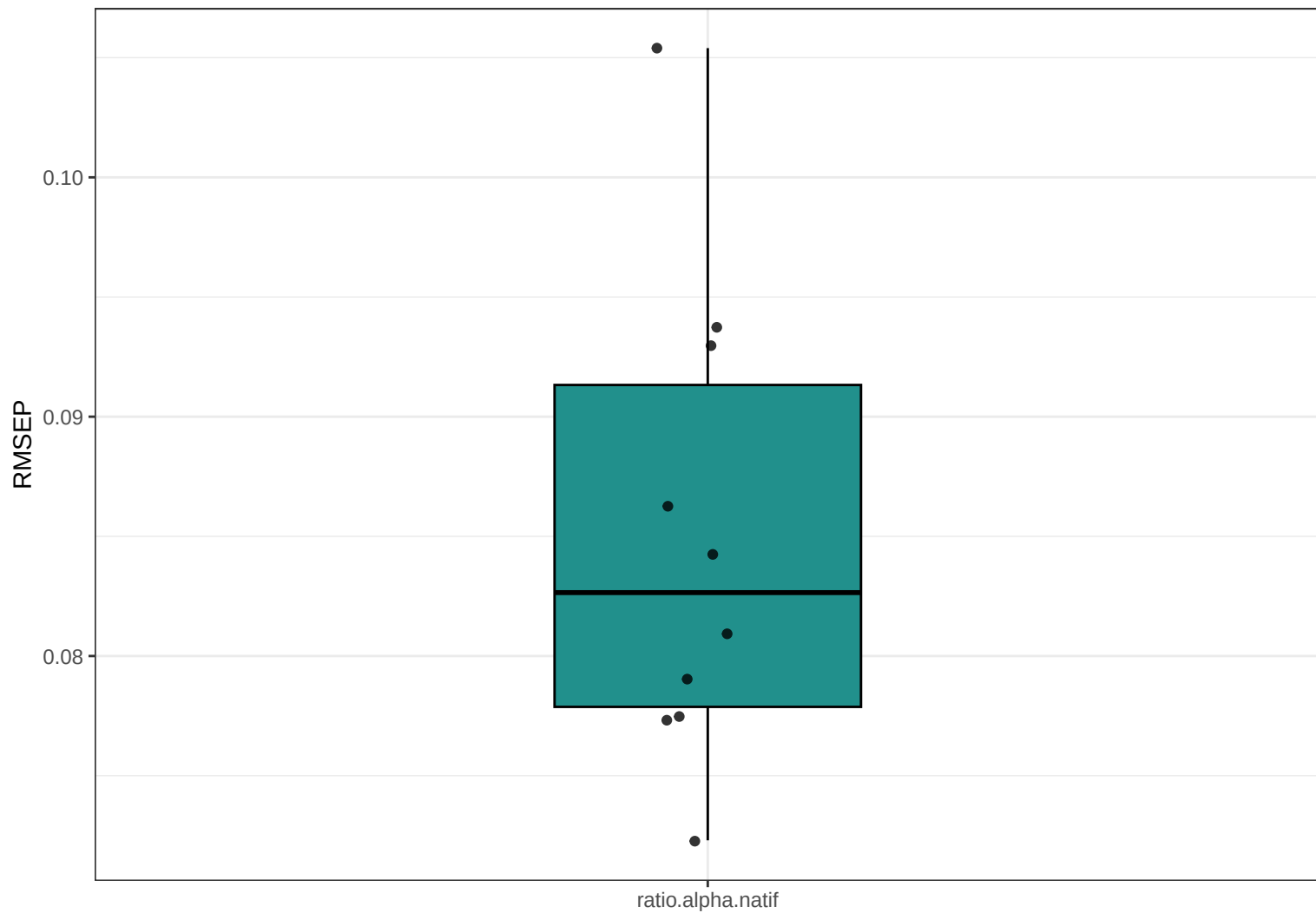
Boxplot RMSEP (PLS) : ratio.alpha.natif
