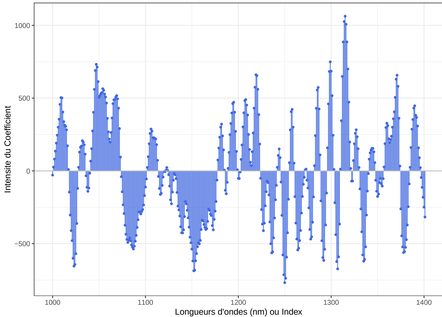
PLS – Vecteur des coefficients : tlip.MS
