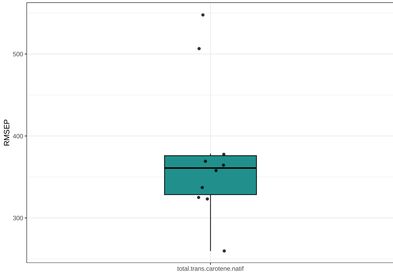
Boxplot RMSEP (PLS) : total.trans.carotene.natif
