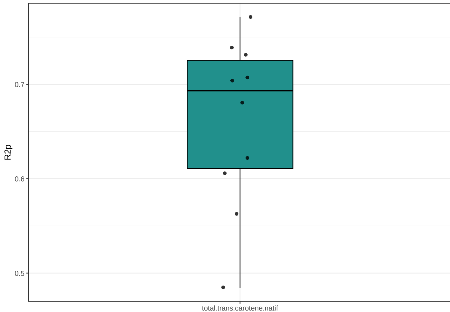
Boxplot R2p (PLS) : total.trans.carotene.natif
