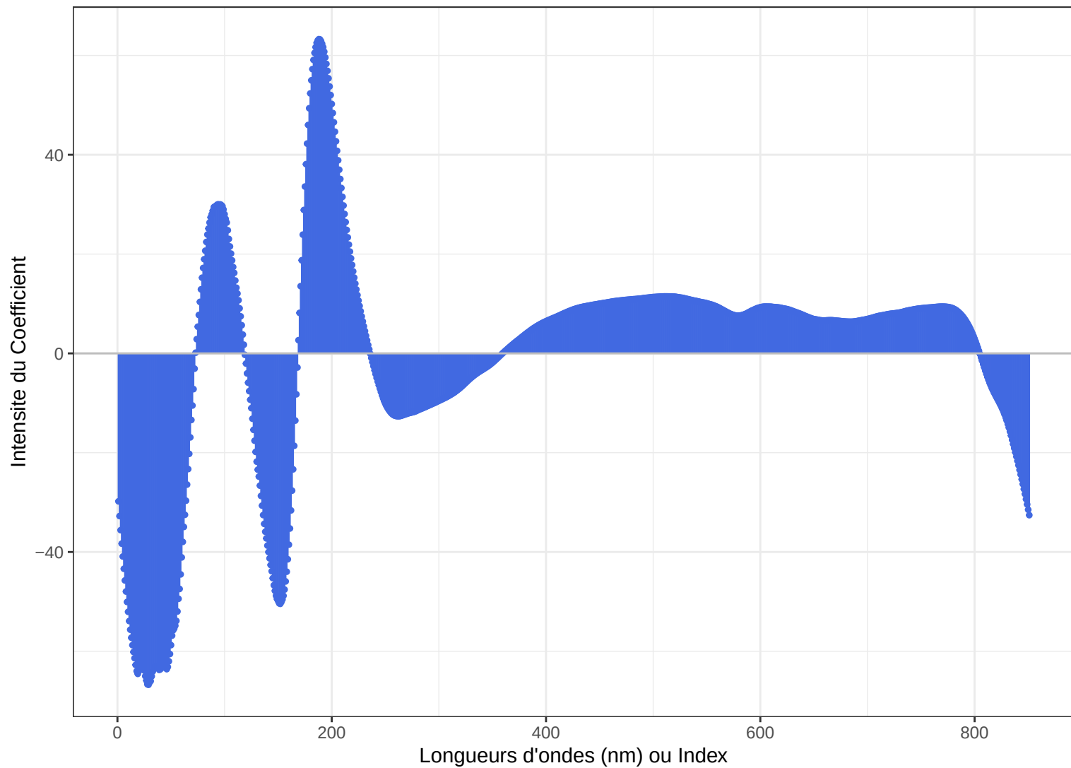
PLS – Vecteur des coefficients : total.trans.carotene.natif
