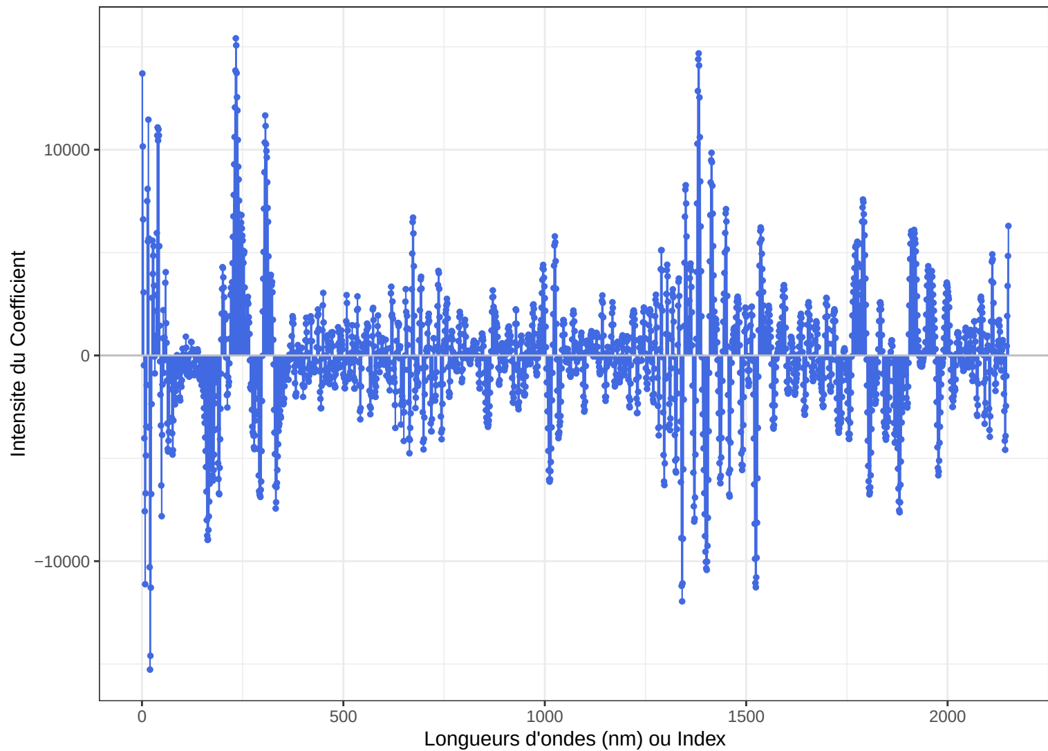
PLS – Vecteur des coefficients : aT
