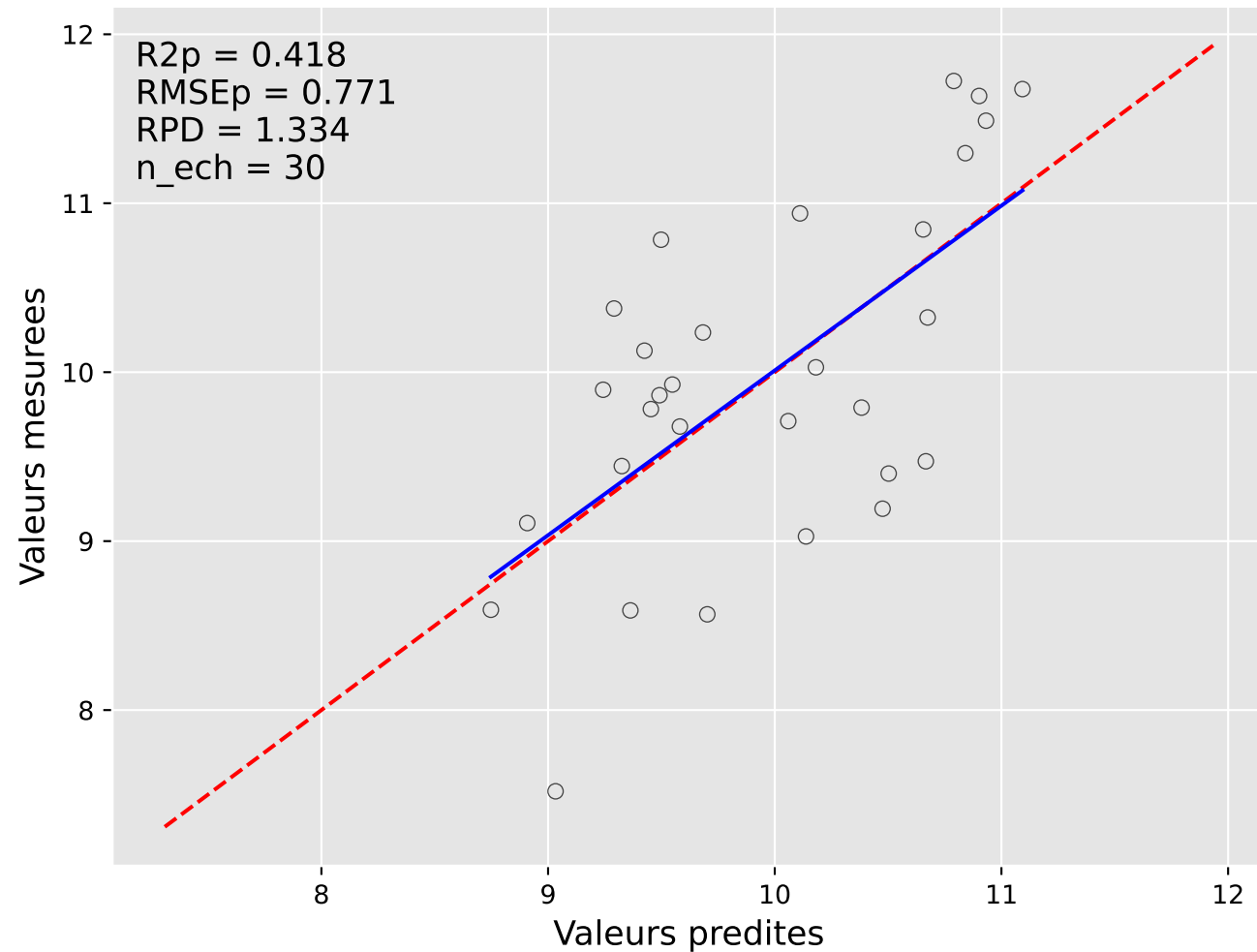
Predictions vs Mesures : C18.2 (lter 2)
