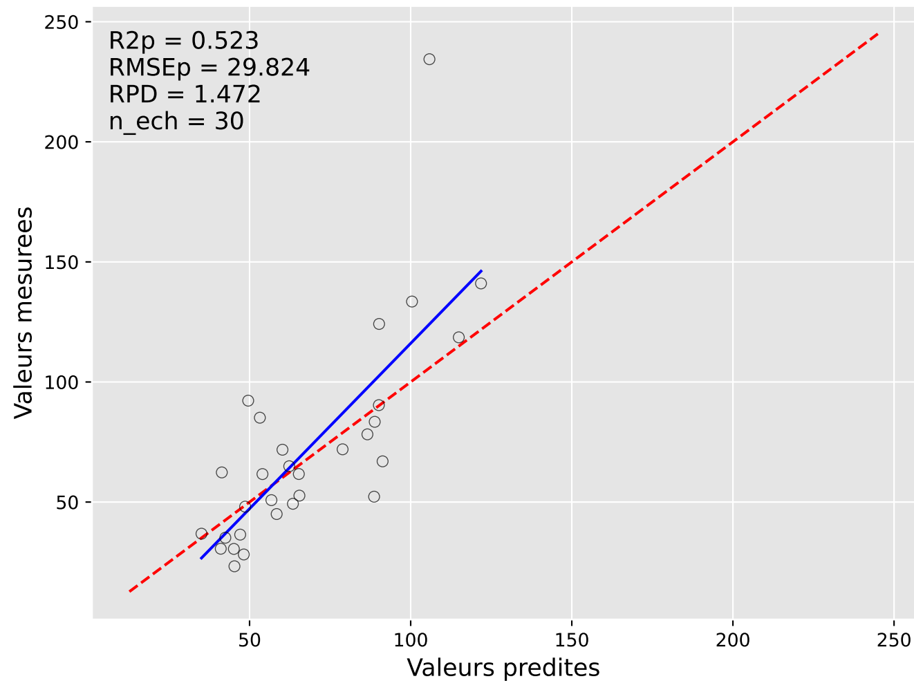
Predictions vs Mesures : X13.cis.beta.carotene (Iter 4)
