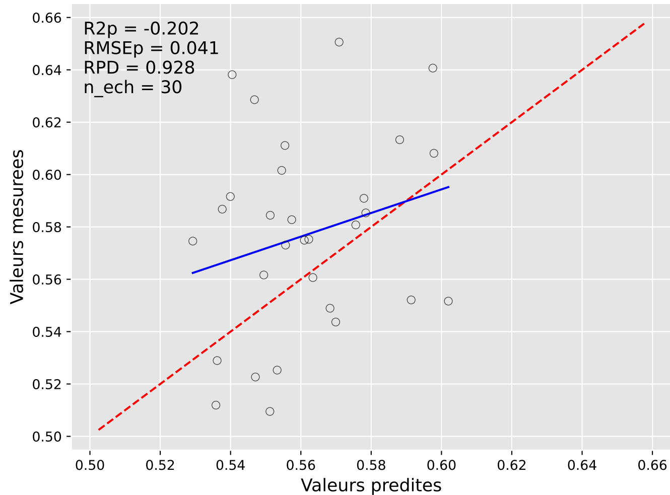
Predictions vs Mesures : ratio.beta.natif (Iter 8)
