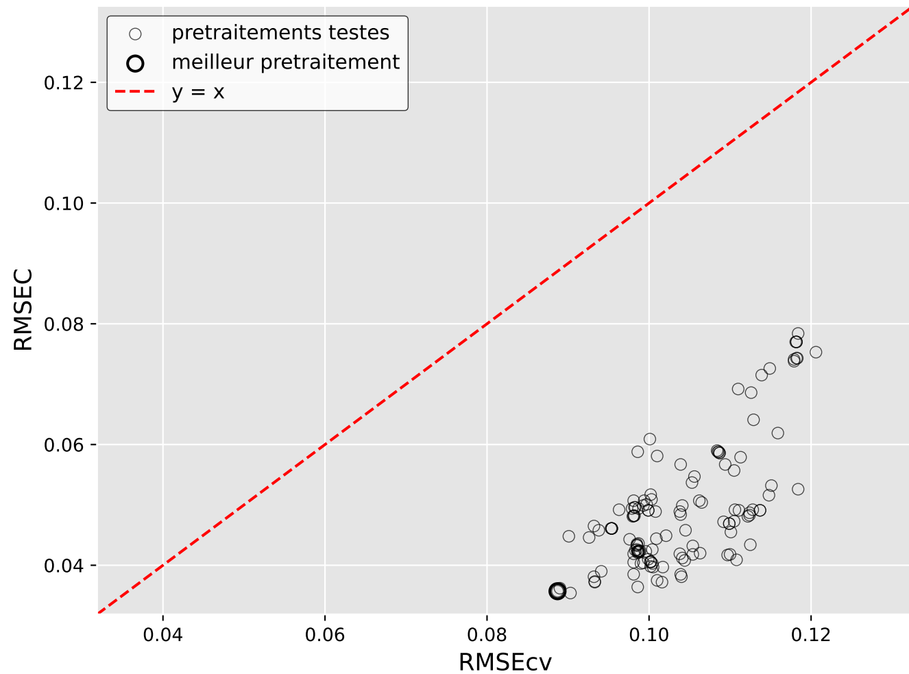
Overfitting pretraitements : ratio.alpha.natif (Iter 5)
