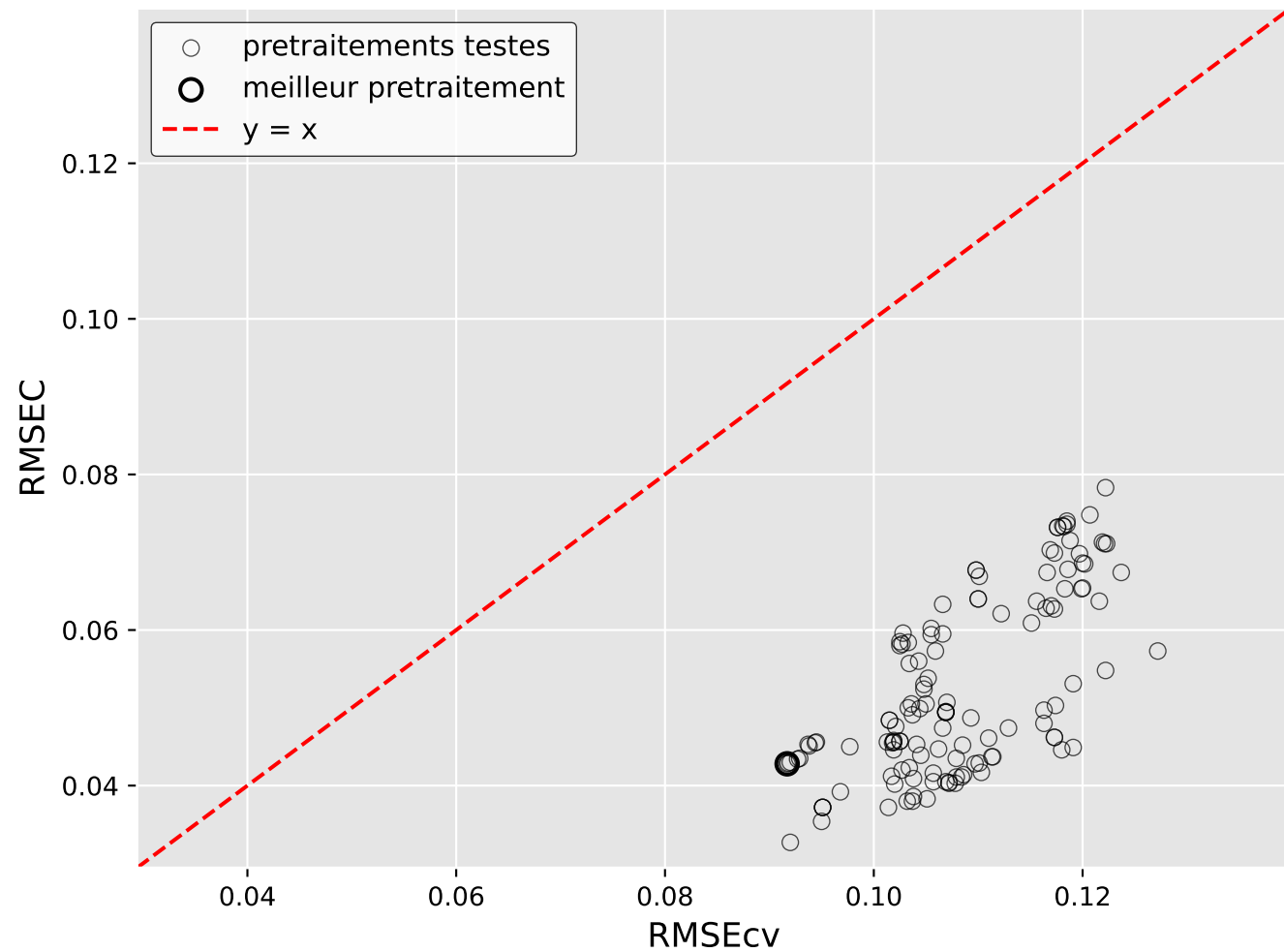
Overfitting pretraitements : ratio.beta.natif (Iter 4)
