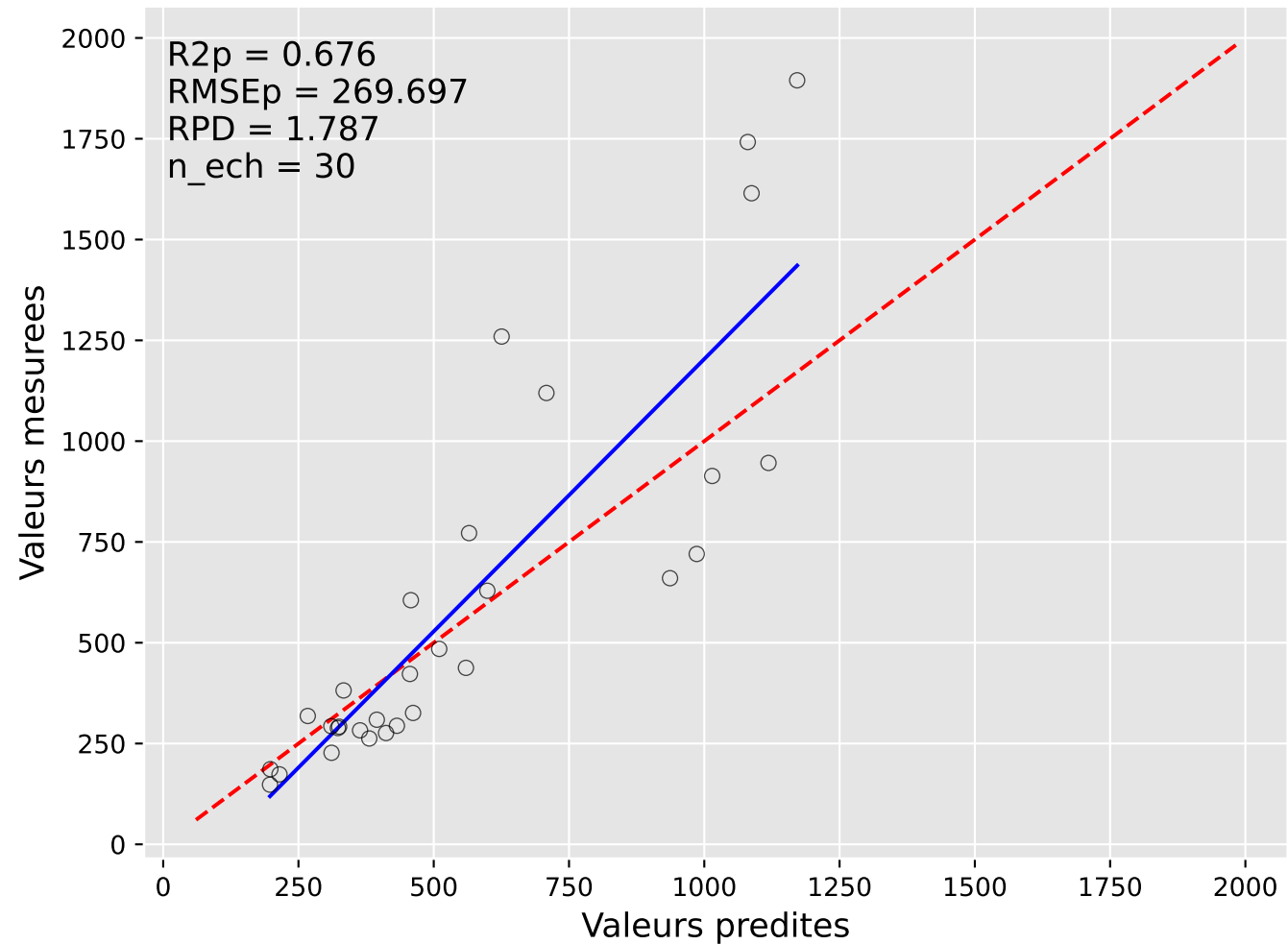
Predictions vs Mesures : total.beta.carotene (Iter 6)
