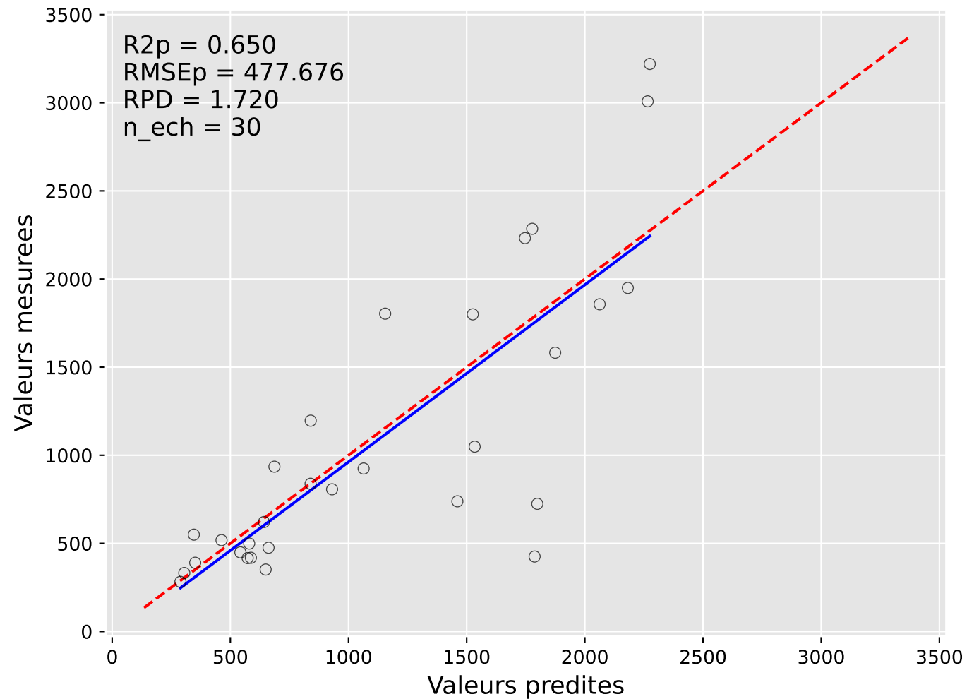
Predictions vs Mesures : total.carotene (Iter 5)
