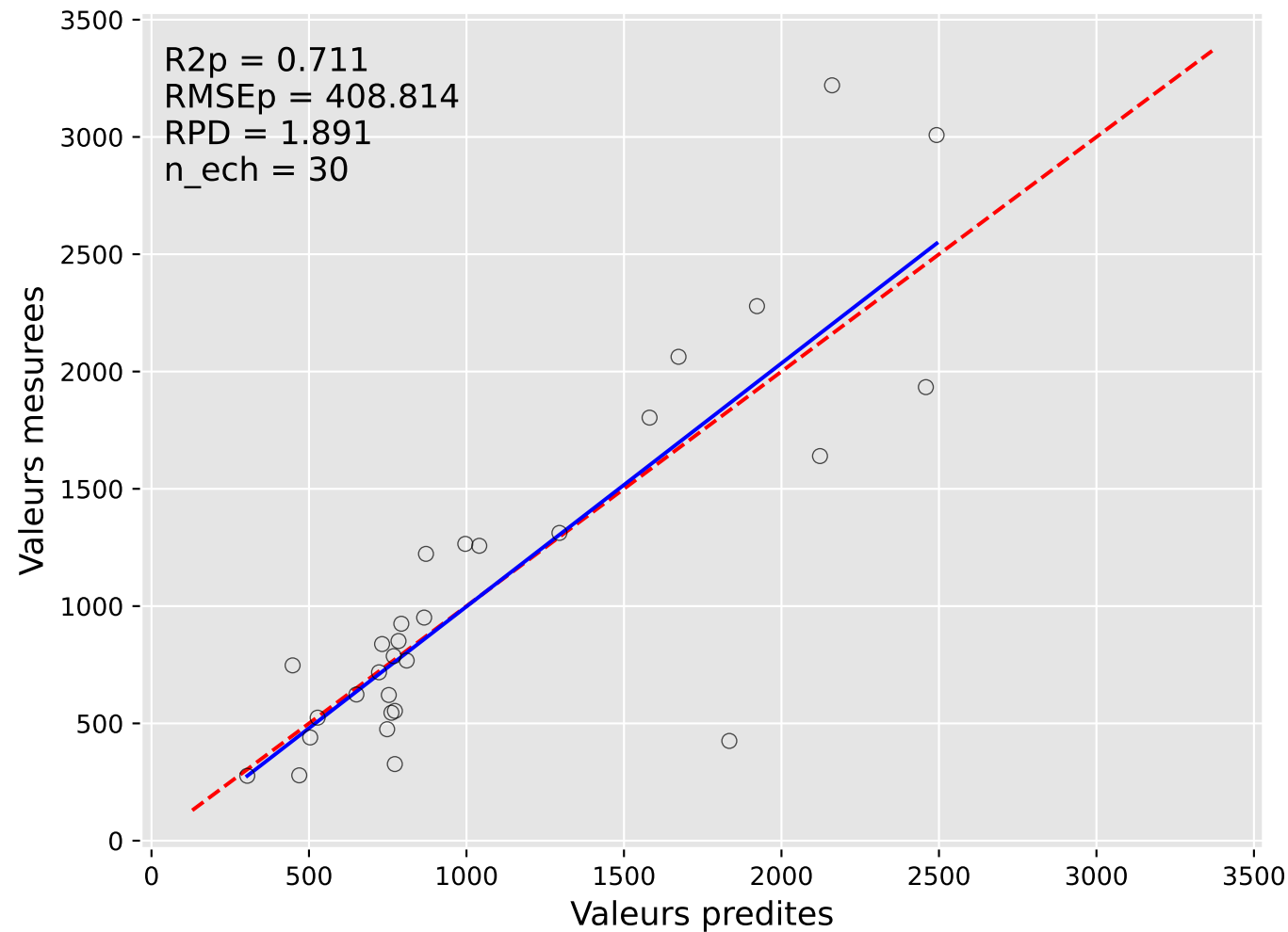
Predictions vs Mesures : total.carotene (Iter 10)
