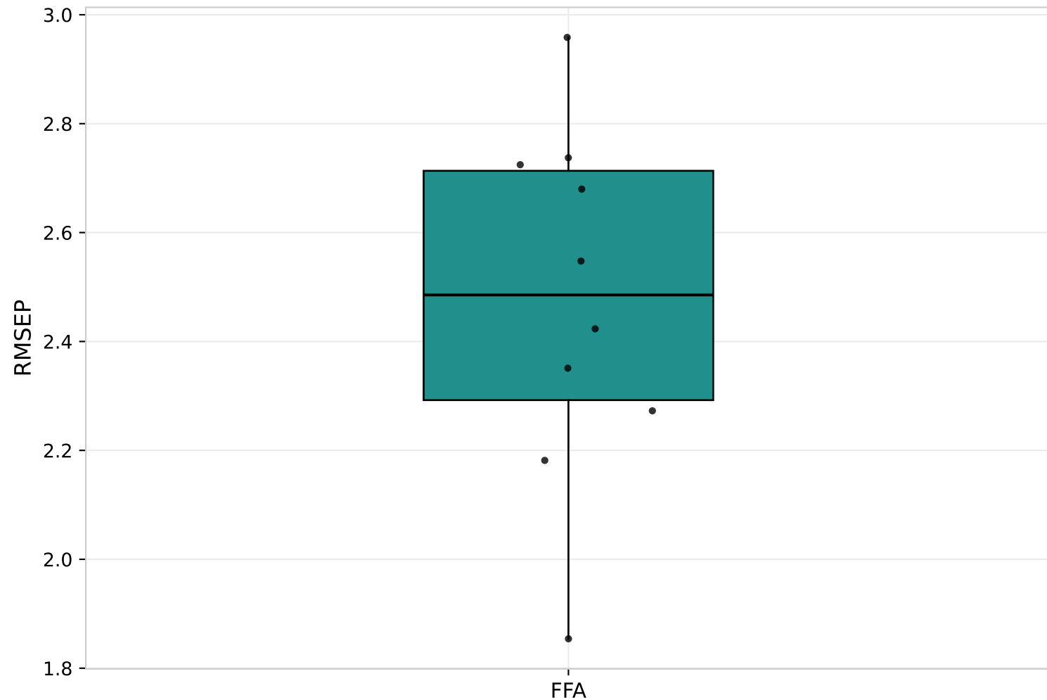
Boxplot des RMSEP obtenus pour FFA sur les 10 iterations
