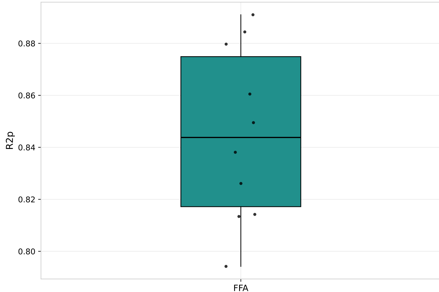
Boxplot des R2p obtenus pour FFA sur les 10 iterations
