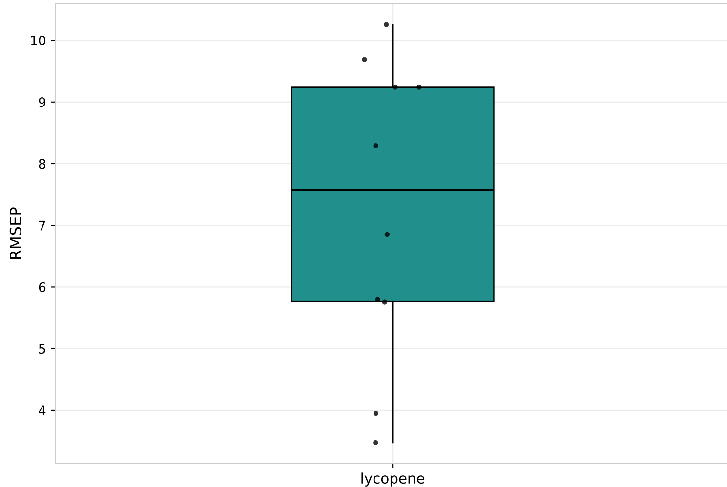
Boxplot des RMSEP obtenus pour lycopene sur les 10 iterations
