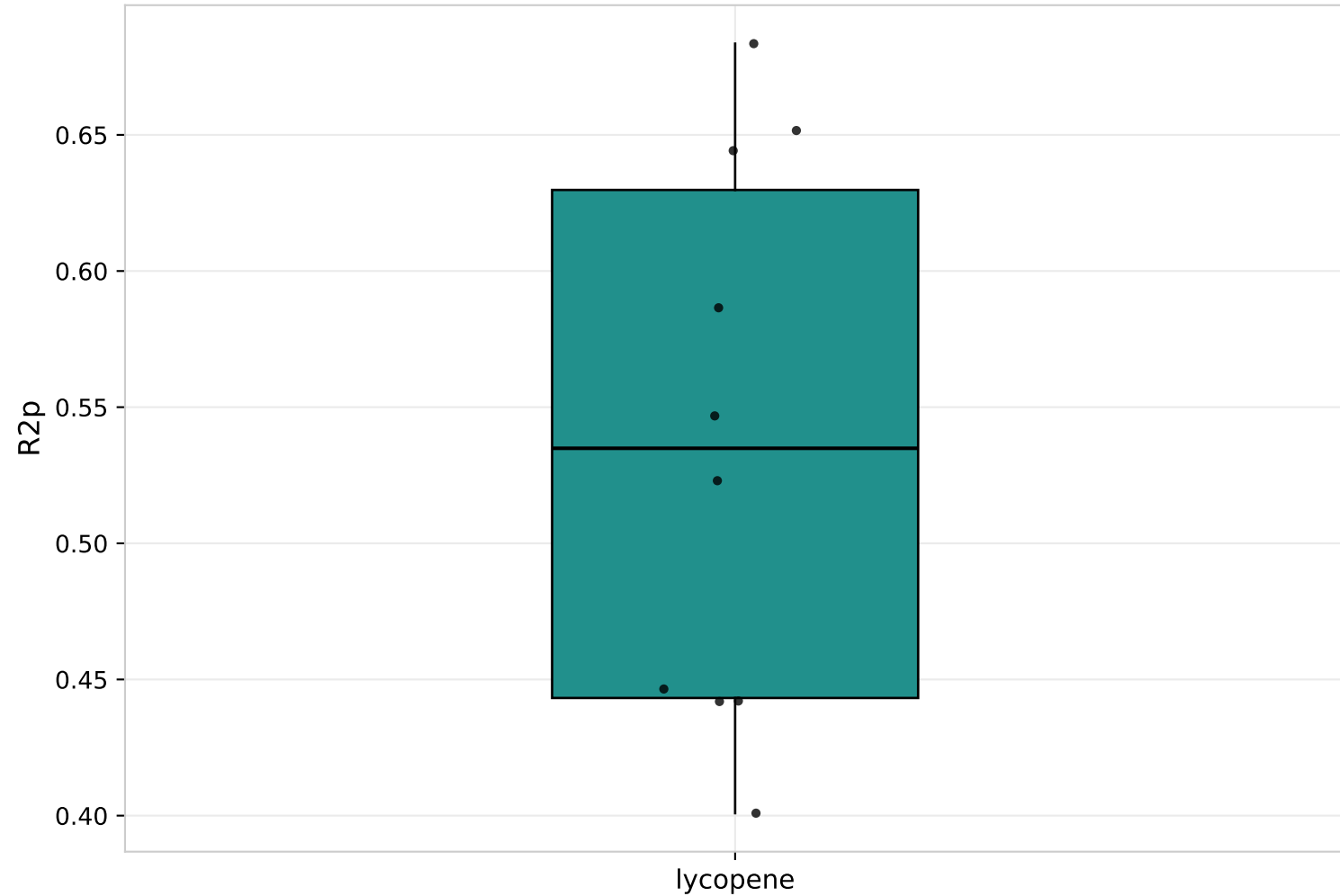
Boxplot des R2p obtenus pour lycopene sur les 10 iterations
